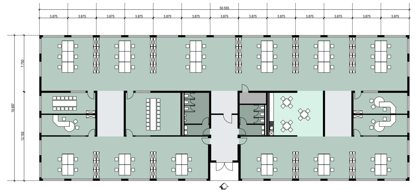
Grundriss Open-Space-Büro
