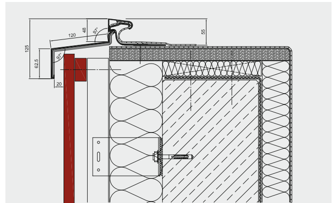
Montage über vorgehängter Holzfassade
