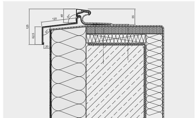
Montage über WDVS
