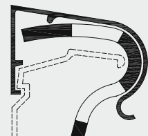
Bitumen-Deckprofil Polymerbitumen-Dachbahn
