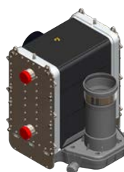
eMAX Hochdruck-Abgaswärmetauscher bis 5.000 Pa
