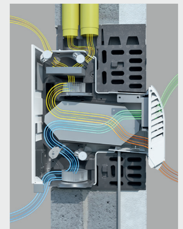
Querschnitt freeAir 100 e mit Kreuzgegenstrom-Wärmetauscher
