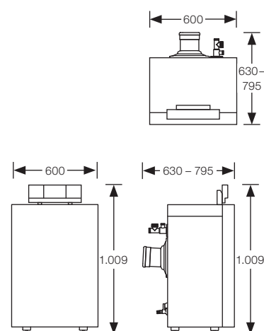
Logano plus KBH192i
