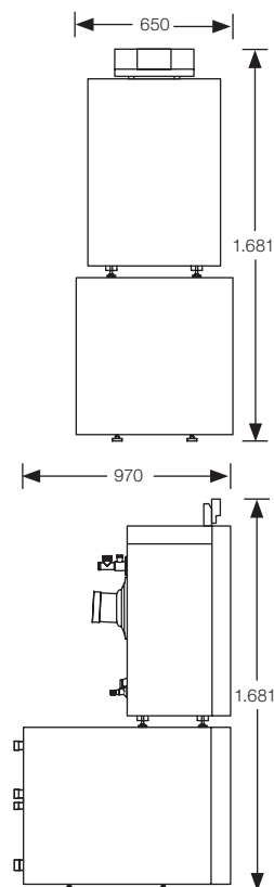
Logano plus KBH192i
