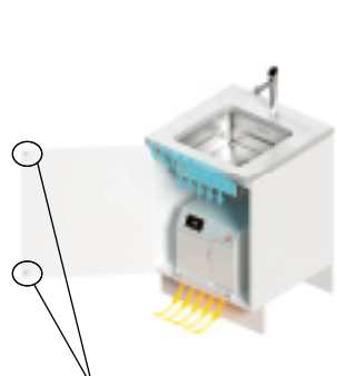
Bei geringer Nutzung reichen für die Zuluft Abstandshalter an der Tür (nicht bei BCS 60 und CS 100)
