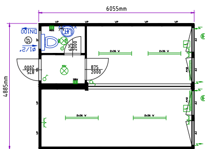
Büro- und Sanitärcontainer 2er-Anlage
