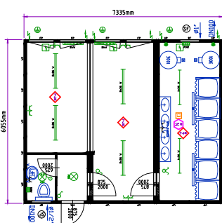
Büro- und Sanitärcontainer 3er-Anlage
