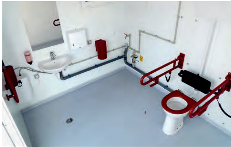
Innenansicht barrierefrei Ausführung nach DIN 18040-1
