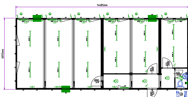
Büro- und Sanitärcontainer 6er-Anlage
