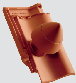
SIGNUM Dunstrohr DN 100 mm mit abschraubbarer Haube
