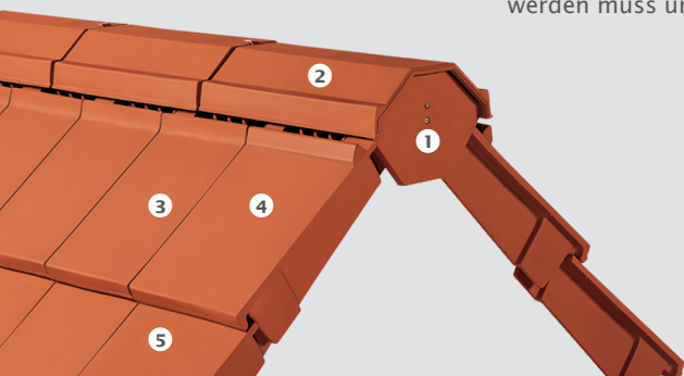
Firstanschluss- Lüfterziegel
