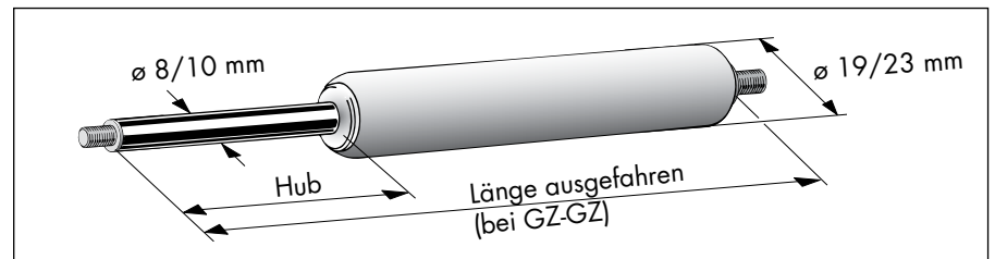
Gewindezapfen GZ
