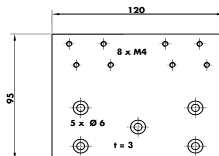
Montageplatte für Türdämpfer V 1600, Bestell-Nr. 205463
