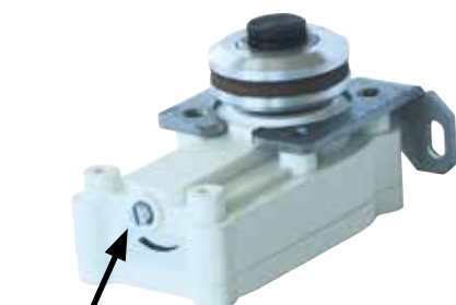
Einstellung Dämpfungskraft (Sechskantschraube mit Schlitz)
