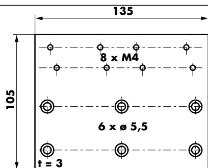
Montageplatte für Türdämpfer VS 2000, Bestell-Nr. 205279
