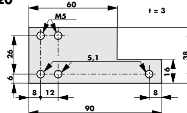
Montagewinkel a für aufliegende Türen, Bestell-Nr. 205220
