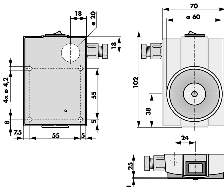
Haftmagnet EM GD 60 F 26 TK
