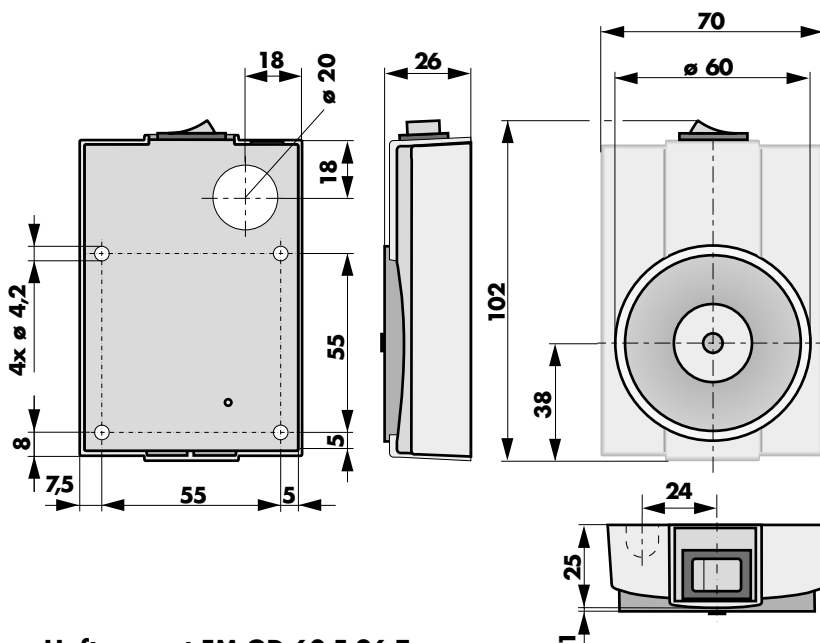
Haftmagnet EM GD 60 F 26 T
