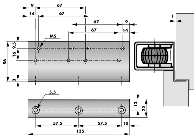
Montagewinkel a für aufliegende Türen, Bestell-Nr. 205220
