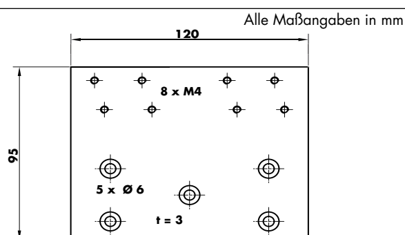
Montageplatte für Türdämpfer V 1600, Bestell-Nr. 205463
