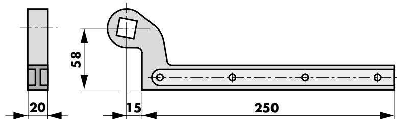
Traghebel 300 (unten) Bestell-Nr. 460086-300
