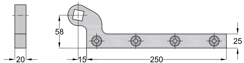
Traghebel 600 (unten) Bestell-Nr. 460086-600
