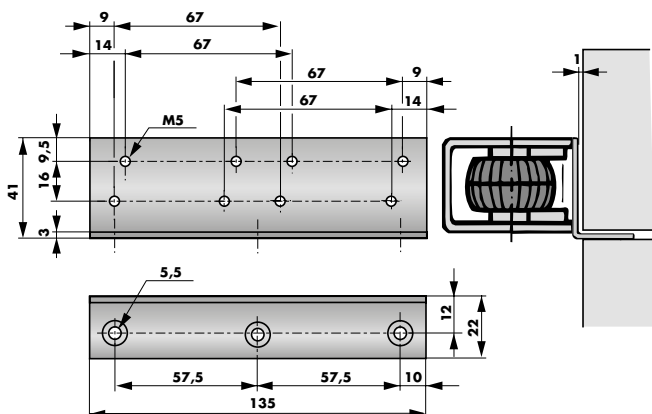
Montagewinkel g für gleichliegende Türen, Bestell-Nr. 205221
