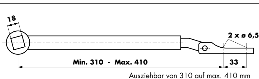
Schiebehebel (unten) Bestell-Nr. 460093
