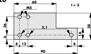
Montagewinkel a für aufliegende Türen, Bestell-Nr. 205220
