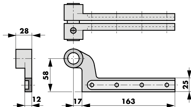
Zapfenband (oben) Bestell-Nr. 460087 bzw. 460094 (mit Nadellager)
