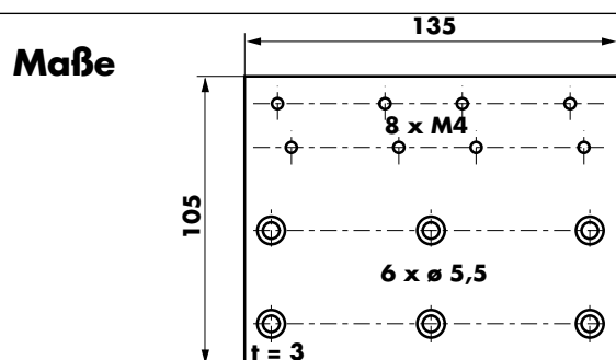
Montageplatte für Türdämpfer VS 2000, Bestell-Nr. 205279
