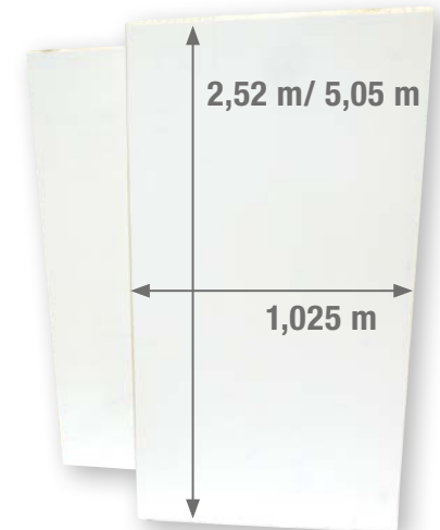
Formate mit 4-Seitiger Nut & Feder/Fase
