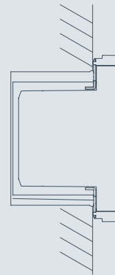
Schematische Darstellung: Corlo Touch KNX in Schalterdose
