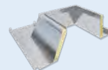
Profil Kranz, Höhe 30 cm
