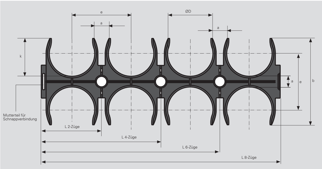
Zeichnung Type 110
