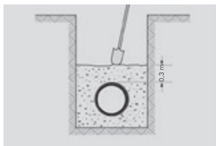
Leitung bis 30 cm über Rohrscheitel mit steinfreiem, verdichtungsfähigem Boden von Hand verfüllen und verdichten
