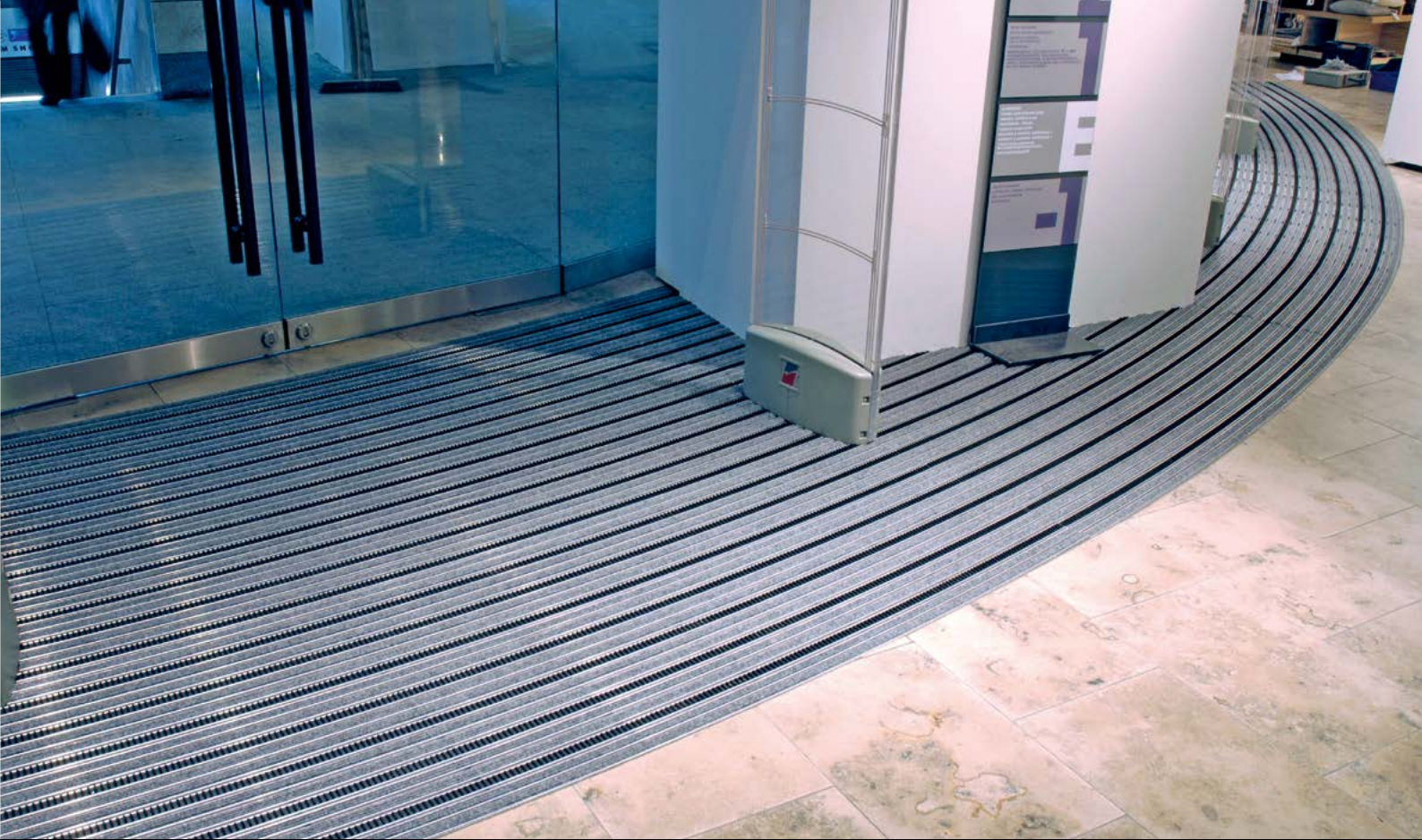
Ludwig Beck Shopping Center, München (Deutschland) Top Clean TREND CURVE 22: Ripseinlage (hellgrau) mit Bürstenprofil (schwarz)
