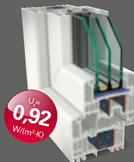
Schmaler Rahmen mit Flügel und bestätigter ift-Passivhaustauglichkeit
