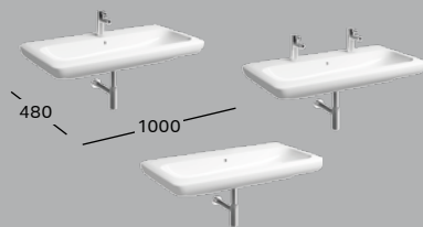
WASCHTISCH B 1000 / T 480 kombinierbar mit Halbsäule Mit Hahnloch, mit Überlauf Ohne Hahnloch, mit Überlauf Mit zwei Hahnlöchern, mit Überlauf
