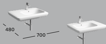
WASCHTISCH B 700 / T 480 kombinierbar mit Halbsäule, mit Hahnloch, mit Überlauf Ablagefläche rechts Ablagefläche links
