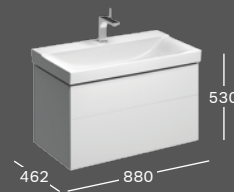
WASCHTISCHUNTERSCHRANK B 880 / H 530 / T 462 1 Schublade, LED-Beleuchtung, optional: Ordnungsboxen für Schubladen Weiß Hochglanz-Lackierung 807290000 Greige Matt-Lackierung 807291000 Holzstruktur Scultura grau 807292000 Melaminharzdekor
