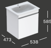
MÖBEL-WASCHTISCHUNTERSCHRANK B 538 / H 585 / T 473
