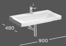
WASCHTISCH B 900 / T 480 ohne Überlauf, Schaftventil mit Ablaufkappe Mit Hahnloch 127090000 Ohne Hahnloch 127093000
