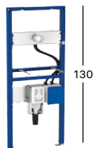
GEBERIT DUOFIX ELEMENT FÜR WASCHTISCH 130 CM Wandarmatur mit UP-Funktionsbox, mit UP-Geruchsverschluss 111.561.00.1
