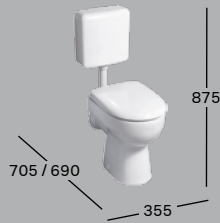
FLACHSPÜL-WC B 355 / H 875 / T 705 / 690 6 l, bodenstehend, freier Zulauf, Abgang waagrecht Flachspül-WC WC-Sitz WC-Sitz mit Absenkautomatik WC-Sitz, antibakteriell Kunststoff-Spülkasten 4,5 / 6 l
