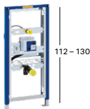
GEBERIT DUOFIX ELEMENT FÜR URINAL 112 – 130 CM universell, für verdeckte Urinal- steuerung 111.689.00.1
