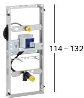
GEBERIT GIS ELEMENT FÜR URINAL 114 – 132 CM universell, für verdeckte Urinal- steuerung 461.689.00.1
