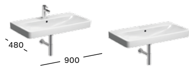
WASCHTISCH B 900 / T 480 Mit Hahnloch, mit Überlauf Ohne Hahnloch, mit Überlauf
