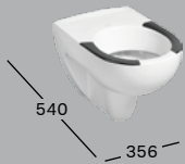
TIEFSPÜL-WC B 356 / T 540 4,5 / 6 l, wandhängend, mit keramischen Sitzflächen Tiefspül-WC
