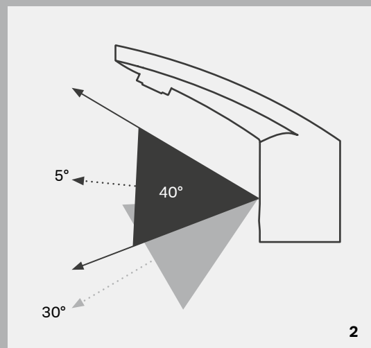
1 Ohne Netz und Batterie: Der Geberit Generator erzeugt Strom aus der Fließkraft des Wassers. 2 Der große Erfassungsbereich des Infrarot-Sensors sorgt für hohe Funktionssicherheit.
