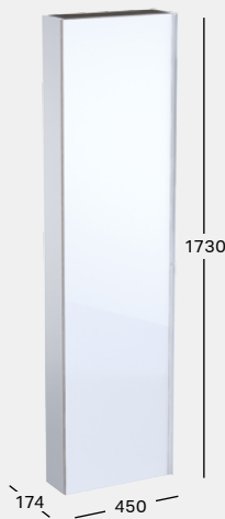
HOCHSCHRANK, FLACH
