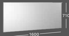
LICHTSPIEGELELEMENT* B 1600 / H 710 / T 55 mit Sensorschalter (dimmbar) und Anti-Beschlag (90 W) Direkte Beleuchtung: 57,2 W, 4095 lm Indirekte Beleuchtung: 51 W, 2940 lm Lichtspiegelement 807360000
