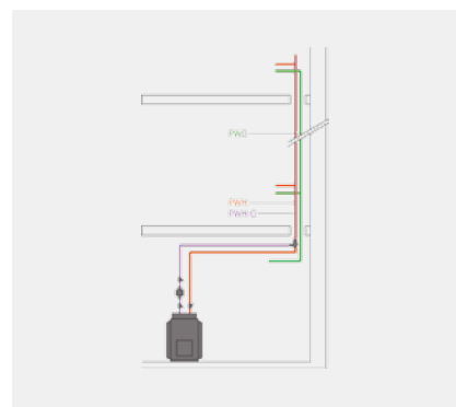
↑ INNENLIEGENDE ZIRKULATION
