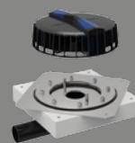
GEberit PLUVIA DACHWASSEREINLAUF mit Befestigungsflansch für Dach- abdichtungsfolien, DN 56
