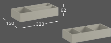
ORDNUNGSBOXEN FÜR SCHUBLADEN B 323 / H 62 / T 150 für alle Waschtischunterschranke und Seitenschränke mit Schublade T-Unterteilung 807910000 Horizontale Unterteilung 807920000
