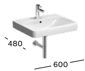
WASCHTISCH B 600 / T 480 Mit Hahnloch, mit Überlauf
