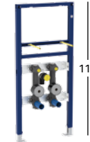
GEBERIT DUOFIX ELEMENT FÜR WASCHTISCH 112 CM Standarmatur, mit zwei Wasserzählerstrecken, UP-Absperrventil und Anschluss-T-Stück
