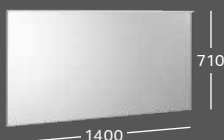
LICHTSPIEGELELEMENT* B 1400 / H 710 / T 55 mit Sensorschalter (dimmbar) und Anti-Beschlag (53 W) Direkte Beleuchtung: 52 W, 3575 lm Indirekte Beleuchtung: 46,6 W, 2660 lm Lichtspiegelement 807340000
