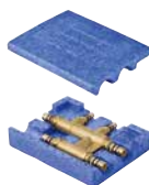
GEBERIT MEPLA KREUZUNGS-T-STÜCK mit Dämmbox, Heizung, DN 12 / 12 / 12 – DN 20 / 15 / 20
