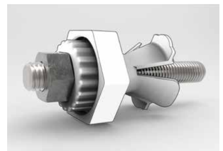
Vormontiertes Schnellmontage-Set
