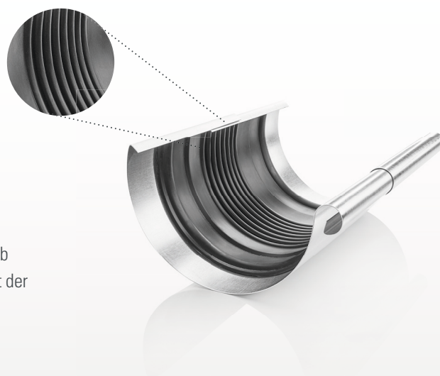
Abbildung zeigt in der Rinne montierte Universal Rinnen-Dilatation inkl. Wulstblende
