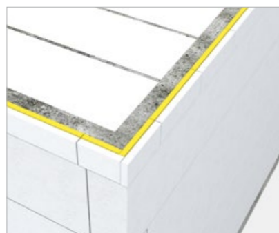
8. Betonieren der U-Schale
