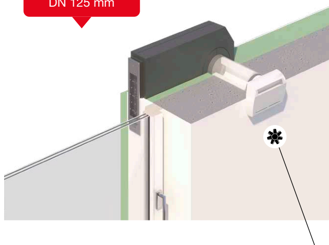
Einbaubeispiel DN 125 mm
