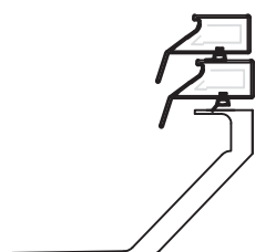
Ausgleichrahmen mit zusätzlichem Lüfterrahmen für Lichtkuppelschalen inkl. Überschlagscharnier und Spindel- oder Elektro- öffner
