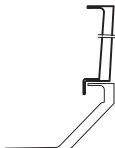
GFK Sanierungskranz SAK mit umlaufender 30-mm- Abkantung zur Montage auf eine waage- rechte Auflage mit mindes- tens 5 cm Breite ( kein neues Eindichten erforderlich )
