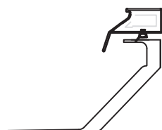
Ausgleichrahmen für starre Lichtkuppelschalen zur Montage auf alle trag- fähigen Aufkantungen
