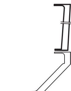
GFK-Sanierungskranz SAK zur Montage auf eine waage- rechte Auflage mit mindes- tens 5 cm Breite ( Eindichten des SAK erforderlich )
