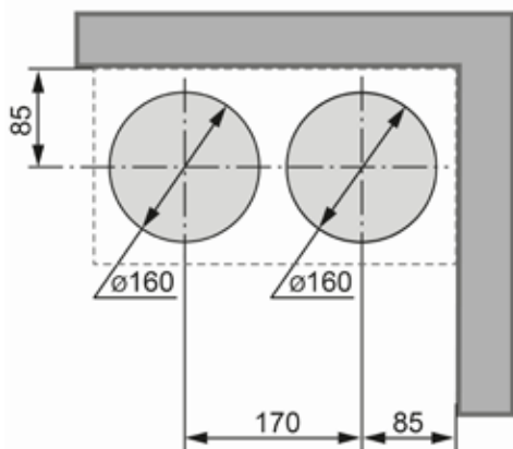
Schema Wandöffnung Außenwand, horizontaler Einbau
