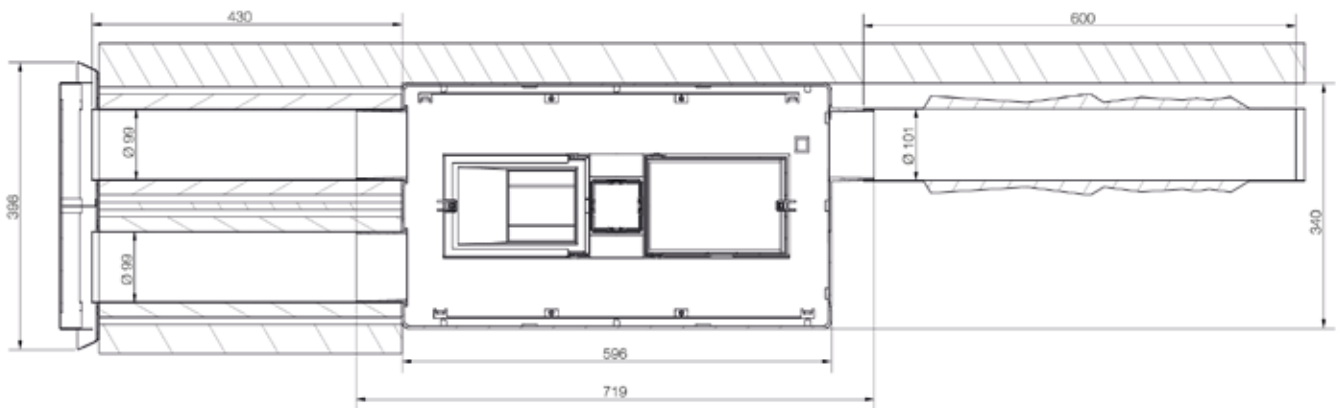
Schema Einbauposition: Einbau an Raumdecke, Ansicht von unten
