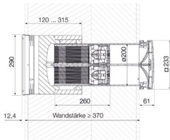
Einbauschema einschaliges Mauerwerk mit Wärmedämmverbundsystem – Draufsicht
