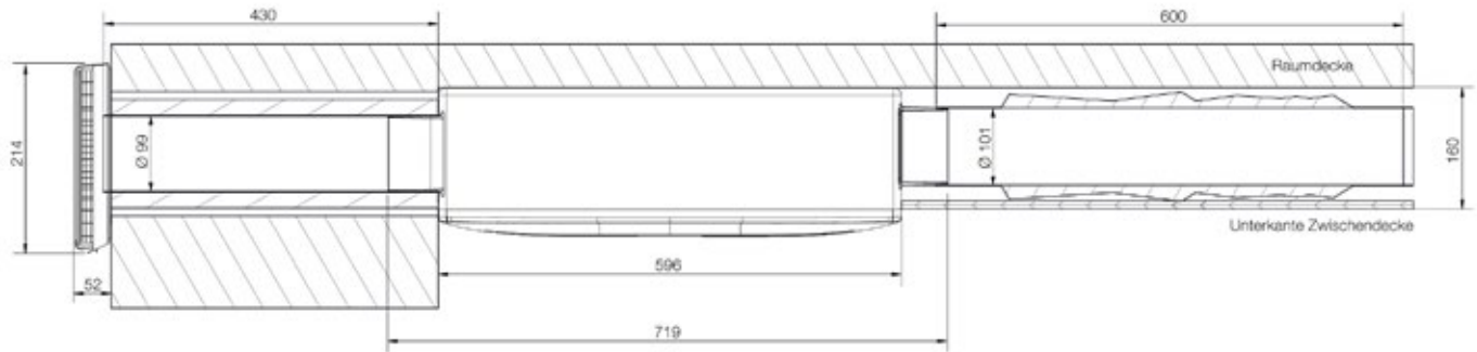
Schema Einbauposition: horizontal in Zwischendecke, Seitenansicht
