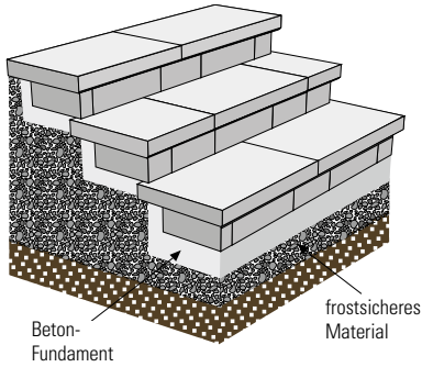
Einbau von Legestufen
