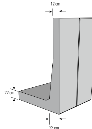
Mauerscheiben Höhe 1,80 m–3,05 m
