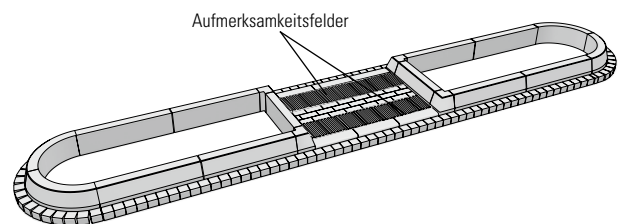
Abb. 26: Mittelinsel mit Nullabsenkung
