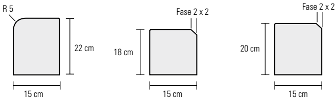
Übergangsstein Anschlussseite Rundbordstein
