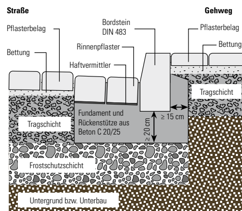
Abb. 12: Einbaueispiel für eine Randbefassung mit einem Hochbordstein aus Beton und Entwässerungsrinne
