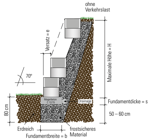
Bei Böschungsbefestigungen mit 70°-Neigung hat es sich bewährt, zwei Pflanzröge übereinander mit doppeltem Versatz aufzubauen. Die entstehenden größeren Pflanzräume lassen die Pflanzen schneller anwachsen.
