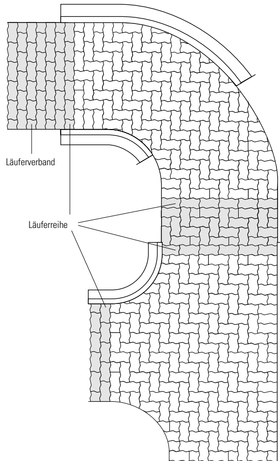
Ausbildung von Kurven und Trompetenstücken im Fischgrätverband
