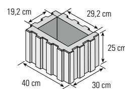
Halbelement
