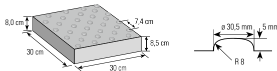
Noppenprofil
