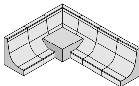
Aufbeton aus Magerbeton C12/15 bei zweiteiligen Winkellecksteinen
