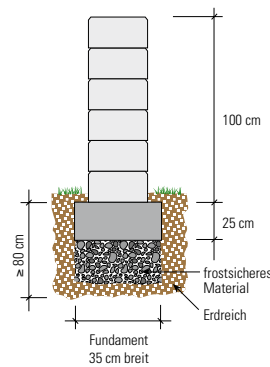
Freistehender Aufbau
