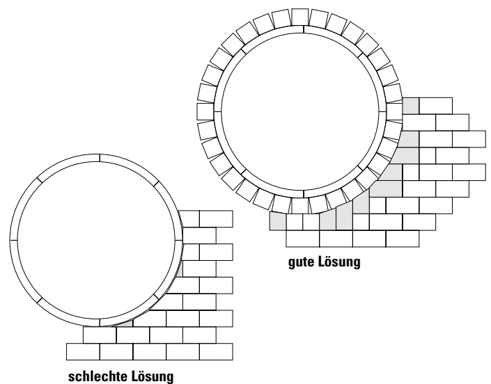
Ausbildung von Kurven und Trompetenstücken im Fischgrätverband
