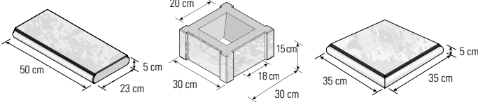
Mauer-Abdeckplatte
