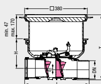
Einbautiefe (T)
