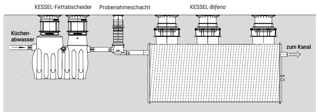
Systembeispiel Bifena zum Einbau im Erdbereich
