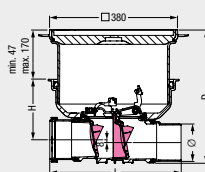
Einbautiefe (T)
