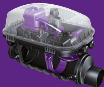
Rückstaupumpanlage Pumpfix F
