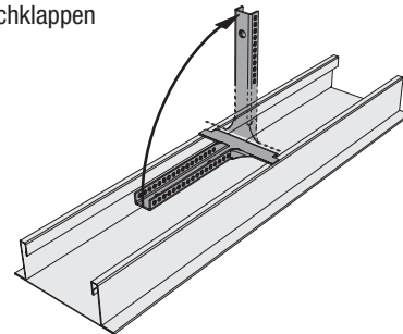
Bild 2.89 - Hochklappen
