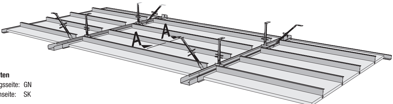
Bild 1.2 - Systemübersicht
