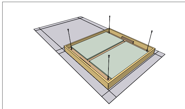
Die beigelegten Seilabhänger an die Basisteile schrauben
