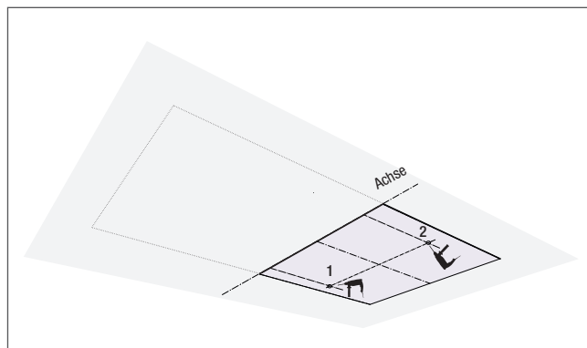
Achse für Deckensegel festlegen. Bohrschablone an Achse anlegen und Bohrlöcher für Abhänger 1 und 2 markieren.
