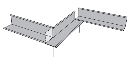
Bild 2.33 - RWL - stumpf
