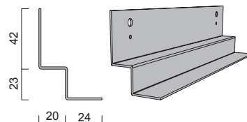
Bild 2.30 - SRW 42/20/23/24 - 3750
