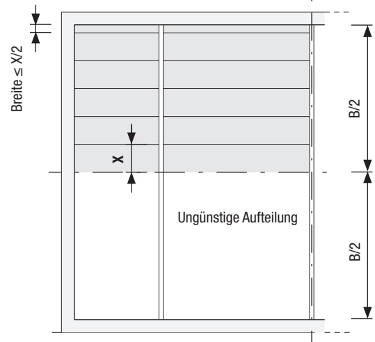
Bild 3.5 Korrektur
