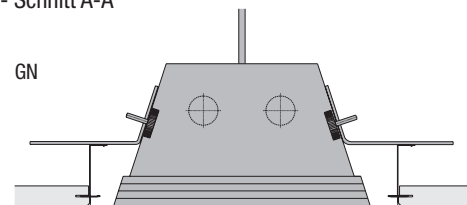
Bild 3.51 - Schnitt A-A
