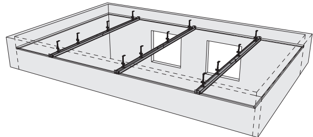
Bild 2.90 - Montage Bandraster
