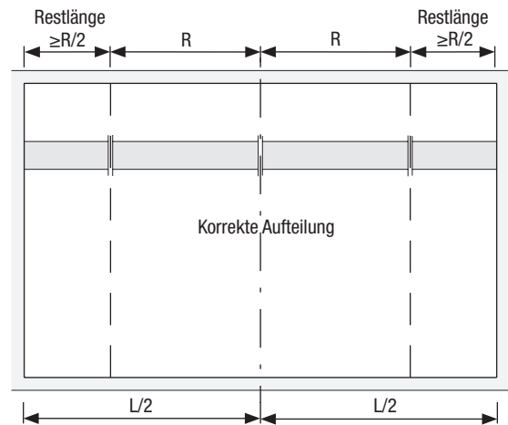
Bild 2.79 - Korrekte Aufteilung
