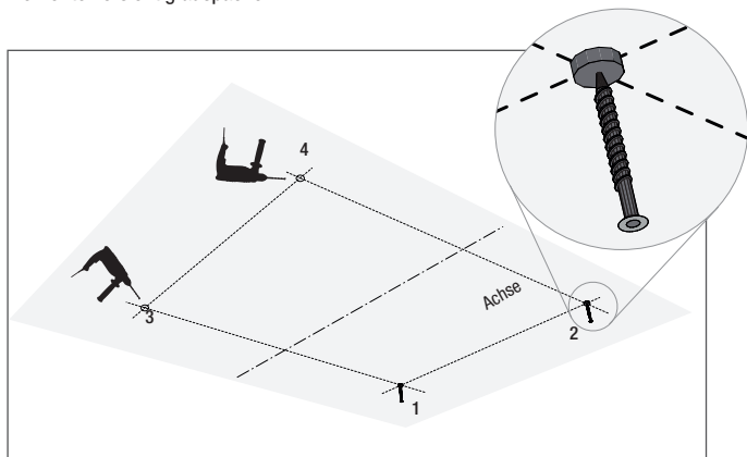
Die Bohrlöcher mit den richtigen Abständen an der Decke anzeichnen und gemäß der verwendeten Befestigungsdübel vorbohren. Die Abhängerobertheile mit für den Untergrund geeigneten Schrauben befestigen.
