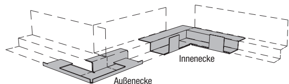
Bild 2.37 - Formteil
