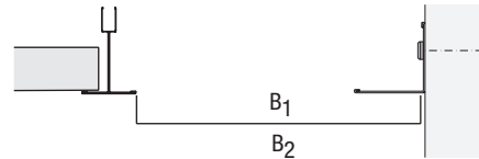
Bild 2.11 - Lichtiges Maß
