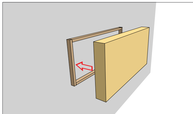
Absorberelement vorsichtig über den Montagerahmen schieben.
