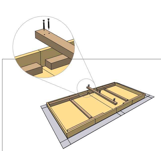
Verbindungsteil C mit 6 Schrauben montieren.
