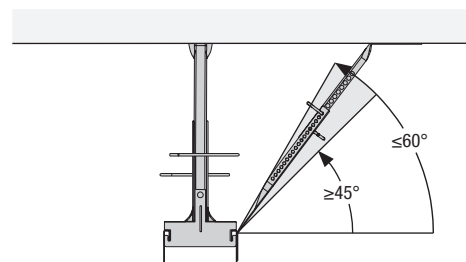
Bild 2.71 - Winkel
