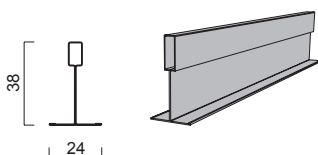
Bild 2.59 - T24/38 - 1800 Kanten GN, AW, SK, VT
