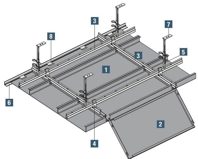
Klemmsystem Langfeldkassette als Klemm-Klapp Variante
