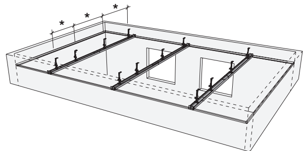
Bild 3.14 Montage Queraussteifung
