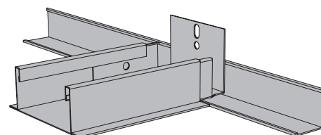
Bild 2.49 - PRB 50-150
