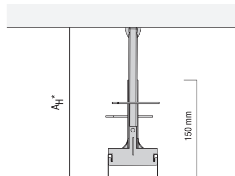
Bild 2.65 - Abhängehöhe
