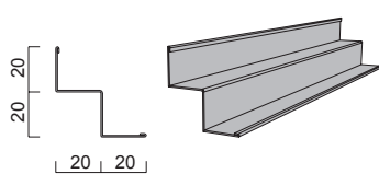
Bild 2.29 - SRW 20/20/20/20 - 3050
