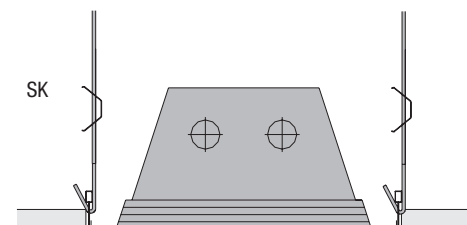
Bild 3.53 - Schnitt A-A
