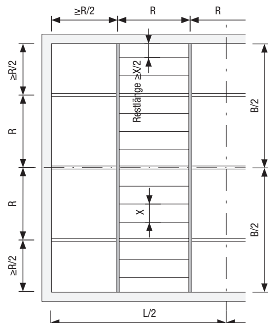
Bild 2.108 - Korrekte Aufteilung
