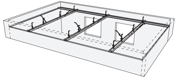
Bild 2.96 - Montage Platten
