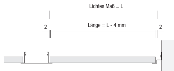
Bild 2.17 - Anschnitt
