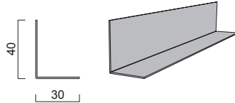
Bild 2.26 - RW L40/30 - 4000
