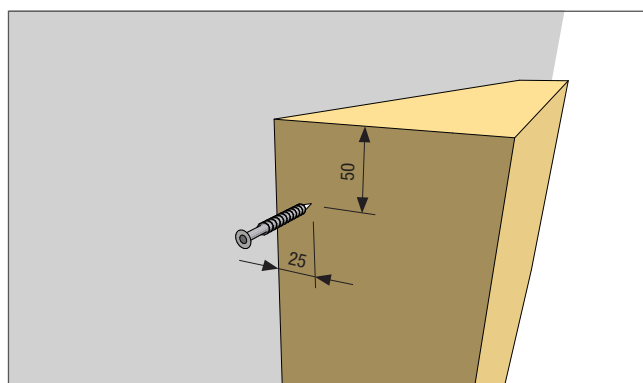
Schraubabstände einhalten!
