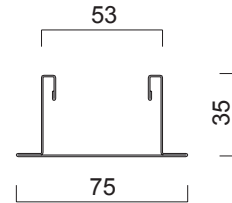
Bild 2.44 - BR 75-3600
