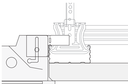
Leuchteinbau CD-Profil
