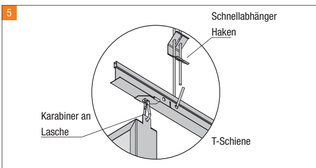
Caddy - Clip an T-Schiene montieren und Baffel mittels Karabiner an Lasche einhängen.
