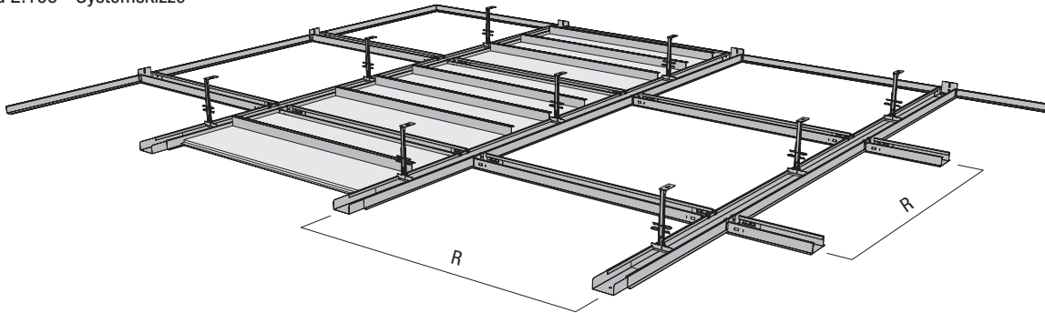
Bild 2.106 - Systemskizze
