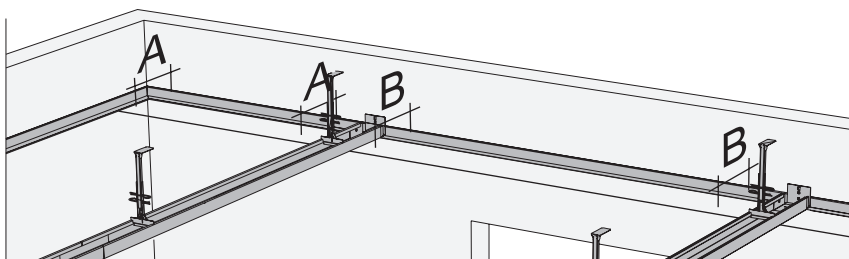
Bild 3.15 - Hilfsmittel Schnur
