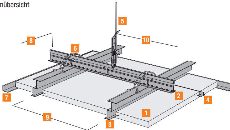
Bild 3.1 - Systemübersicht
