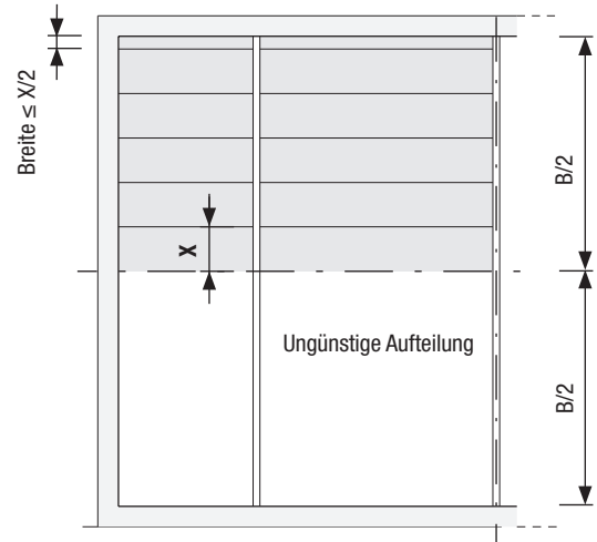
Bild 2.82 - Korrektur
