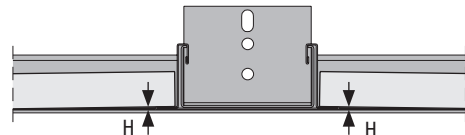
Bild 2.51 - Wandanschluß
