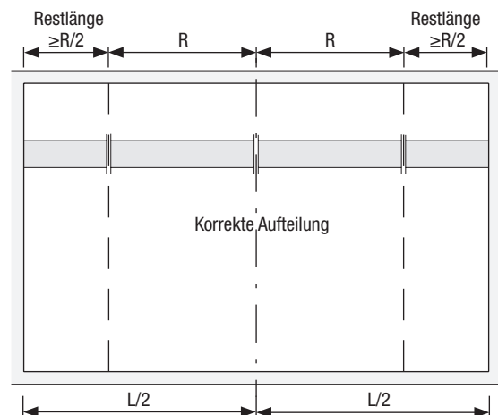
Bild 3.2 Korrekte Aufteilung
