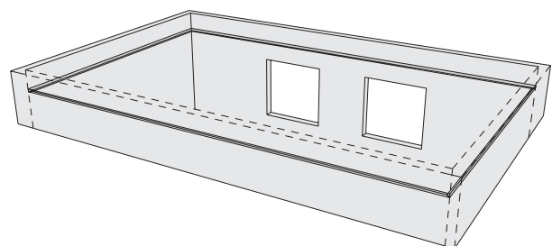
Bild 3.8 - Montage Randwinkel
