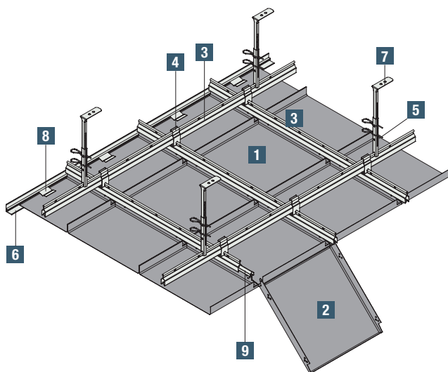
Klemmsystem Quadratkassette als Klemm-Klapp Variante
