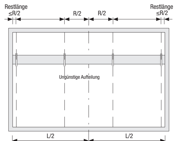
Bild 3.3 Ungünstige Aufteilung
