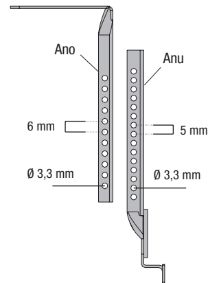
Bild 2.66 - Lochteilung
