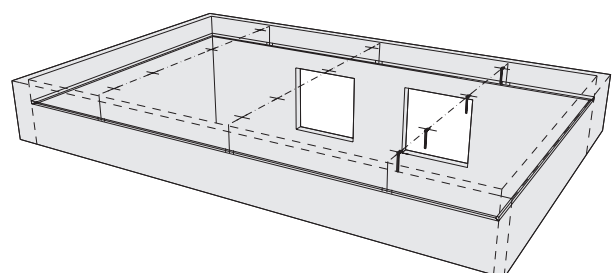
Bild 3.10 - Abhänger
