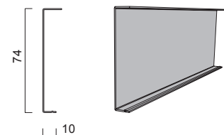
Bild 2.58 - P U10/74/17 - 2500 Kante GN
