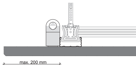
Indirekte Beleuchtung (Rand) CD-Profil
