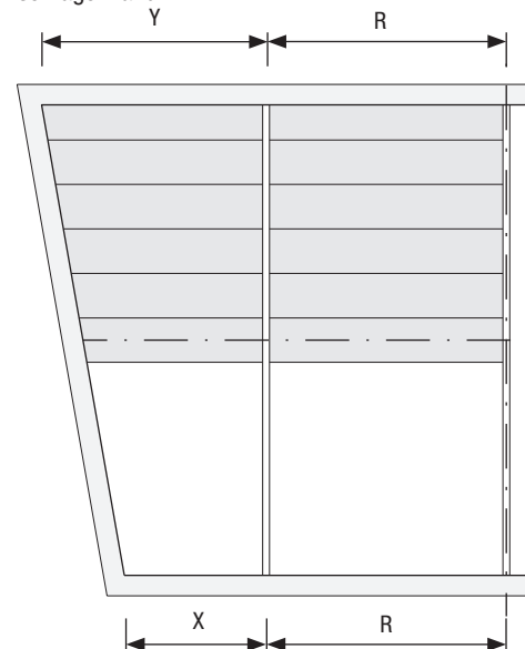
Bild 2.83 - schräge Wand
