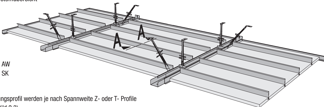
Bild 2.2 - Systemübersicht
