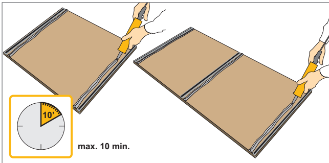
Auftragen von 2 bzw. 3 Kleberaupen HERADESIGN® connect. Durch die vorgefertigte Düse wird ein dreieckförmiger Auftrag des Klebers gewährleistet. Durchschnittlicher Verbrauch: ca. 1 Kartusche pro ca. 1,5 m 2 (basierend auf Plattenformat 1200 x 600 mm)
