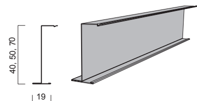
Bild 2.61 - P Z19/40, 50, 70 - 2500 Kanten GN, AW
