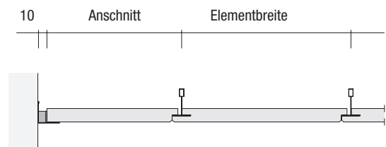
Bild 2.101 - Spaltmaß
