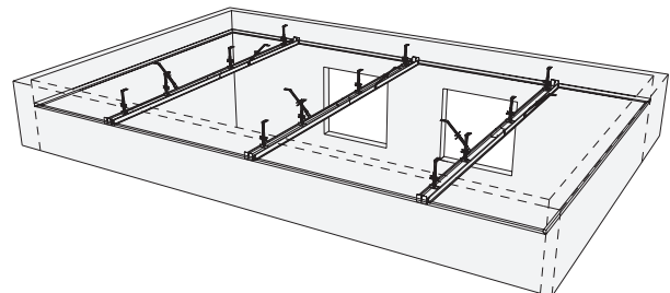
Bild 2.91 - Montage Queraussteifung
