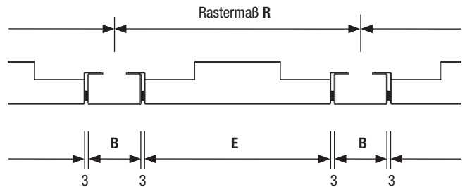
Bild 3.1 Raster
