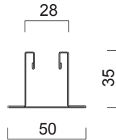
Bild 2.43 - BR 50-3600
