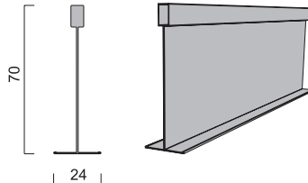
Bild 2.60 - DXE 24ZG - 2500 Kanten GN, AW, SK, VT
