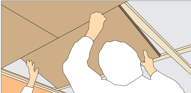
Anbringen der Platten auf Holzlatten oder CD-Profilen (innerhalb von 10 Minuten). Mindestquerschnitt der Holzlatten 60 x 30 mm. ACHTUNG! CD-Profile Standardbreite: 60 mm.
