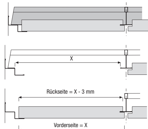
Schnitt B-B
