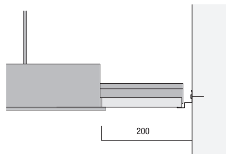
Bild 3.47 - Schnitt B-B
