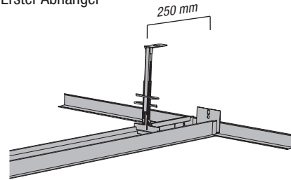
Bild 2.68 - Erster Abhänger
