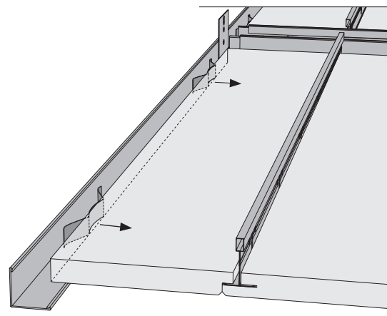
Bild 2.102 - Anordnung
