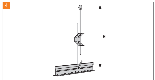
Die Abhänger sind grundsätzlich senkrecht zu montieren. Der maximale Abstand der Abhänger ist vom Reihenabstand der Baffeln abhängig. Anschließend die T-Schiene einhängen.
