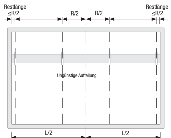
Bild 2.80 - Ungünstige Aufteilung
