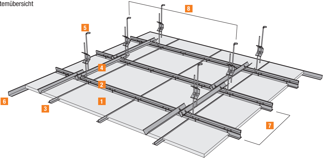
Bild 2.1 - Systemübersicht
