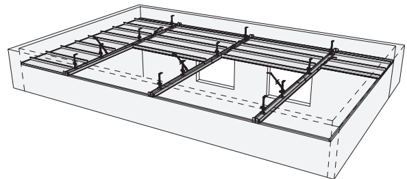
Bild 2.96 - Montage Platten
