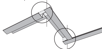
Bild 2.36 - SRW - stumpf
