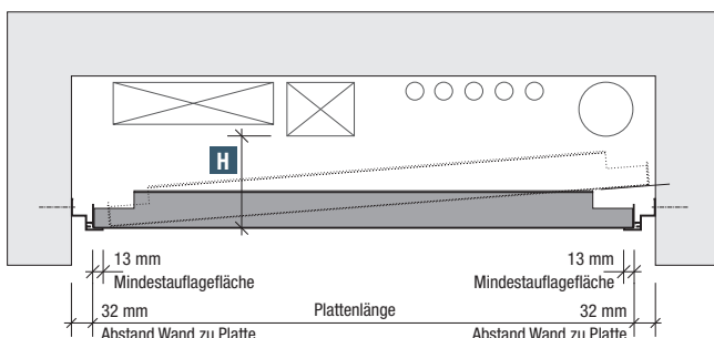
Bild 4.10 - Variante SRW-Stufenrandwinkel
