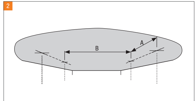
Die Abstände in Längs- und Querrichtung sind auf die gewünschte Befestigungsposition zu übertragen.
