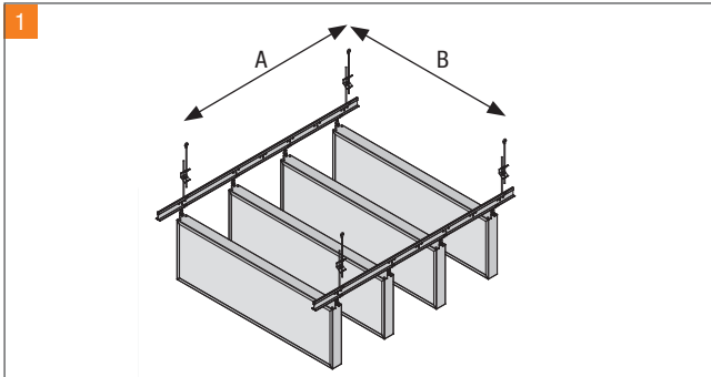
Montage mittels Caddy - Clip und Karabiner an Lasche
