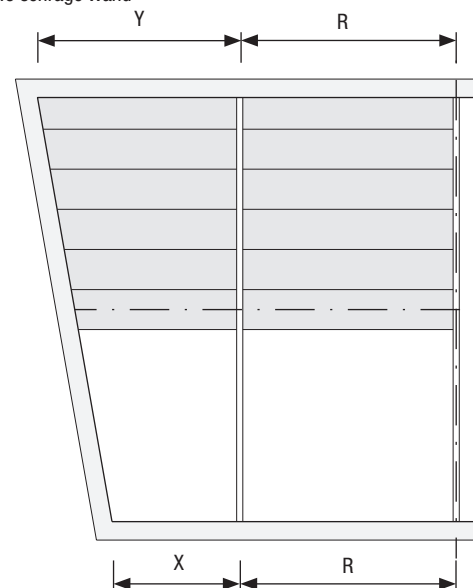
Bild 3.6 schräge Wand
