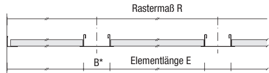
Bild 2.78 - Raster
