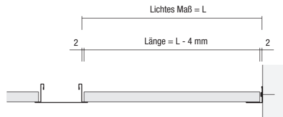
Bild 2.16 - Anschnitt
