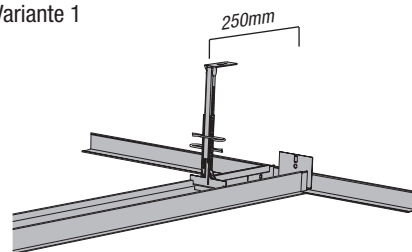
Bild 2.52 - Variante 1
