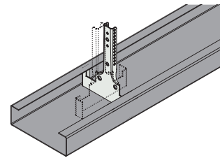
Bild 3.13 - Montage Bandraster
