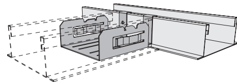
Bild 2.108 - Korrekte Aufteilung
