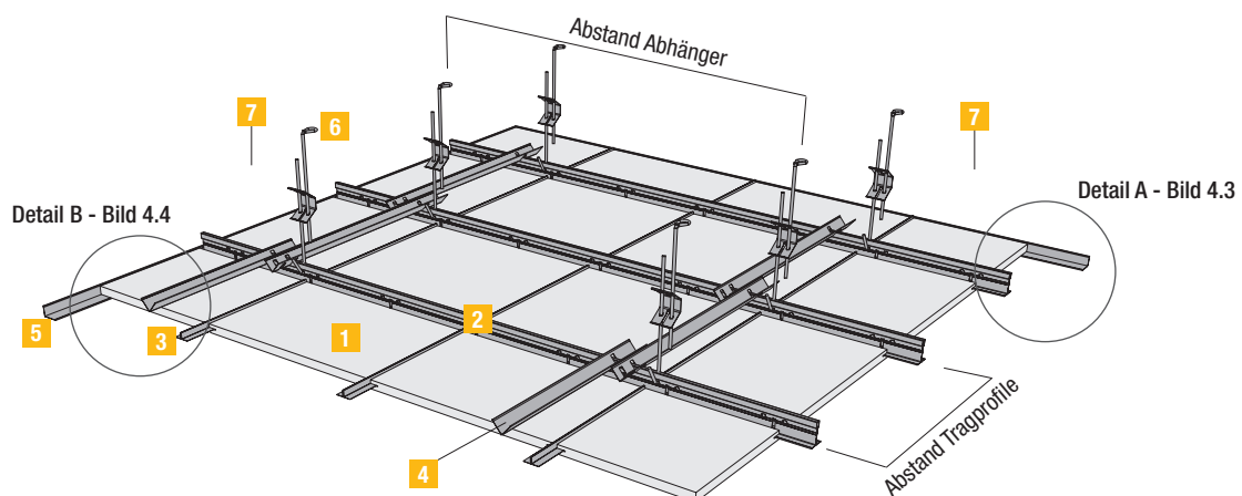
Bild 4.1 - Systemübersicht
