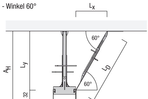
Bild 2.73 - Winkel 60°
