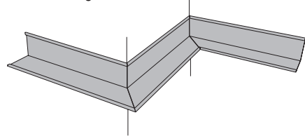
Bild 2.32 - RWL - Gehrung
