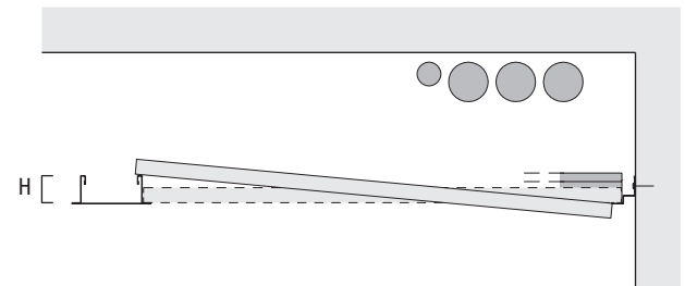
Bild 2.77 - Bandraster - Randwinkel
