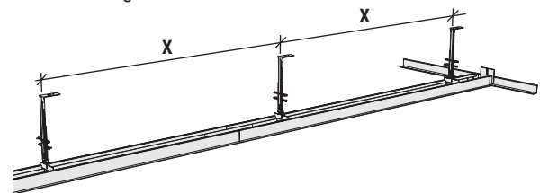
Bild 2.69 - Abhängerabstände
