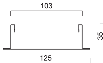
Bild 2.46 - BR 125-3600
