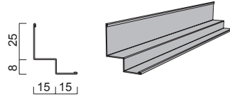
Bild 2.27 - SRW 25/15/8/15 - 3000
