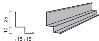
Bild 2.28 - SRW 25/15/10/15 - 3000
