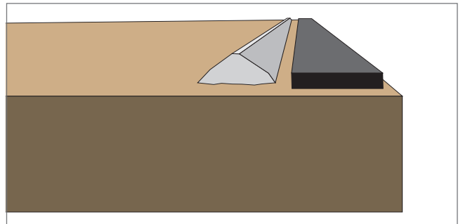
Es ist wichtig auf genügend Abstand zwischen dem Kleber und dem Tape zu achten (ca. 3 mm). Direkter Kontakt zwischen diesen 2 Komponenten ist zwingend zu vermeiden (Verlust der Ersthafung!).
