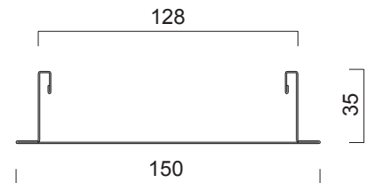
Bild 2.47 - BR 150-3600
