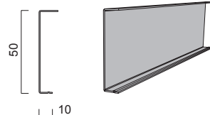
Bild 2.57 - P U10/50/17 - 2500 Kante GN
