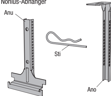
Bild 2.64 - Nonius-Abhänger
