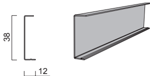
Bild 2.56 - P U12/38/12 - 2000 Kante GN
