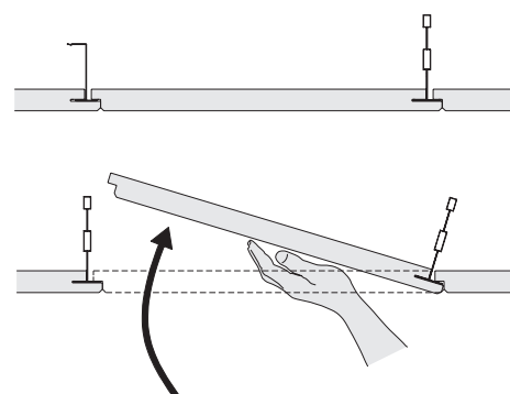
Bild 2.3 - Schnitt A-A, herausnehmbar
