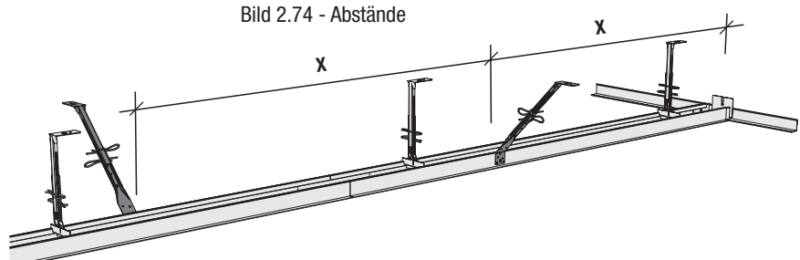
Bild 2.74 - Abstände
