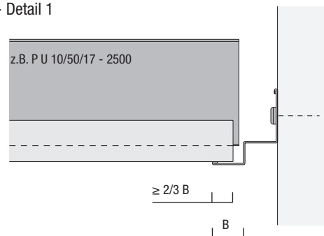
Bild 1.6 - Anwendung 1
