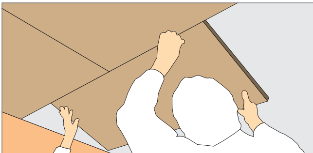
Anbringen der Platten auf Beton (innerhalb von 10 Minuten). Exaktes Ansetzen und Anpressen der Akustikplatten. Ausfluchten der Plattenreihen mit Verlegeplatte.
