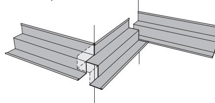
Bild 2.35 - SRW - stumpf
