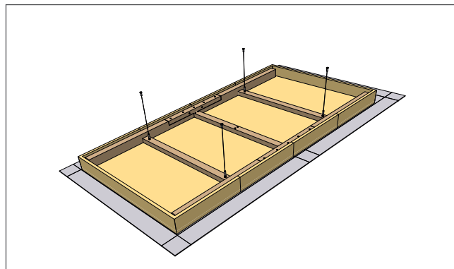
4 Stk. Abhänger montieren
