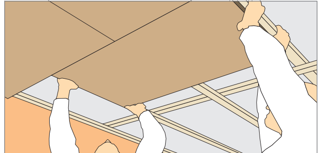
Exaktes Ansetzen und Anpressen der Akustikplatten. Ausfluchten der Plattenreihen mit Verlegeplatte, Plattenstöße müssen mittig unter dem Profil angeordnet sein. Auf eine plane Plattenoberfläche ist zu achten. Ein nachträgliches Ausrichten der Platten ist nicht mehr möglich.
