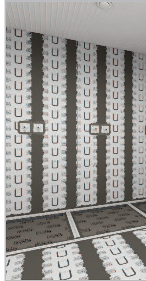
Duschbereich mit bahnenförmiger Abdichtung
