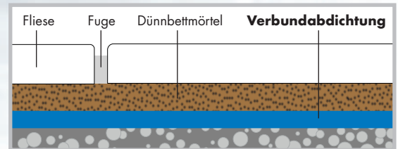
Schema Fliesenverbundabdichtung
