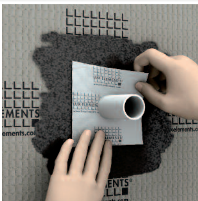
LUX ELEMENTS®-DRY-DBWM Dichtmanschette mit vorgefertigtem Loch für Abdichtung von Rohrdurchführungen
