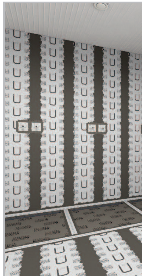
Duschbereich mit bahnenförmiger Abdichtung
