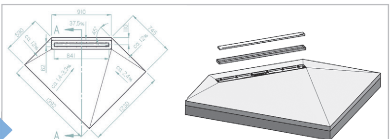
Duschboden mit Linienentwässerung TUB-LINE PLUS Individuelle Maßanfertigung
