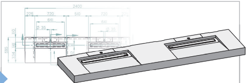
Waschtisch LAVADO PLUS Individuelle Maßanfertigung
