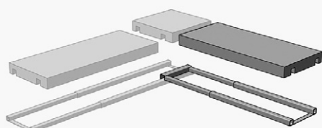
Bankform FLOAT – Eckausbildung von Wand zu Wand gerade, inkl. Edelstahlunterkonstruktion
