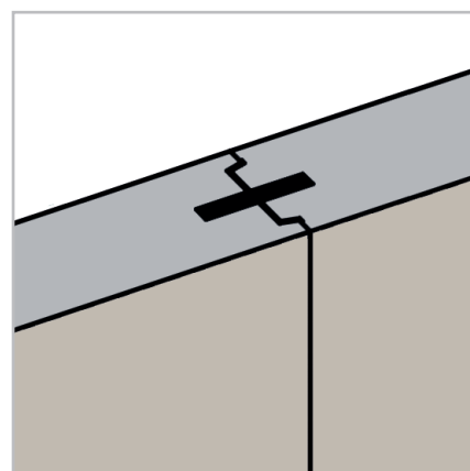
Plattenverbindung aus Feder und V-Fräsung
