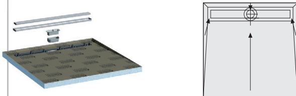
TUB-LINE Q4 ... – quadratisch / 4-seitiges Gefälle
