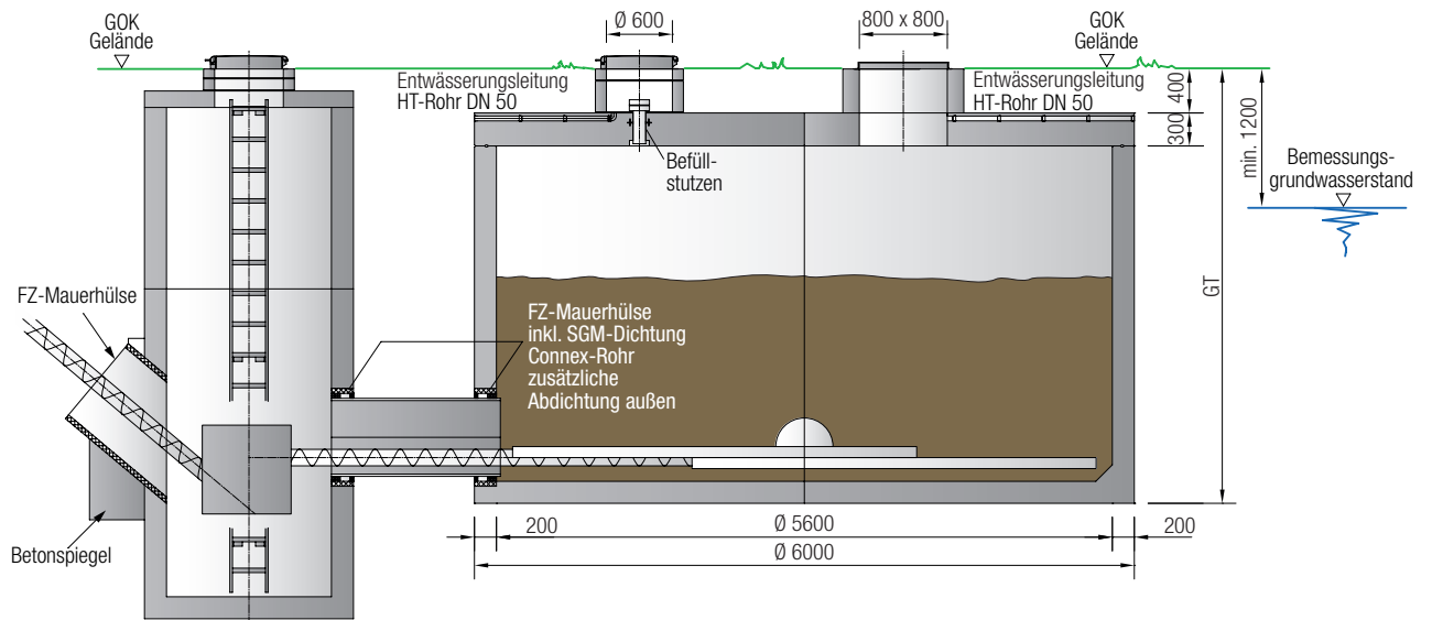
Mall-Revisionsschacht rund
