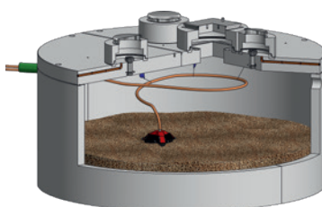
Mall-Pelletspeicher mit Maulwurf 6000 - E3
