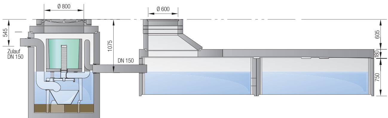
Substratfilter ViaPlus
