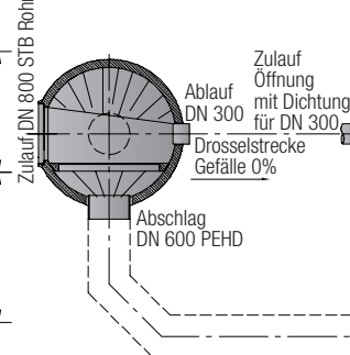
Trennbauwerk ViaSep
