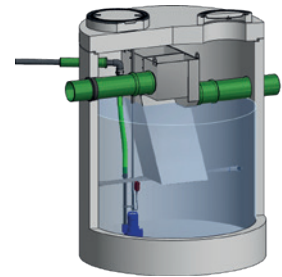
Mall-Lamellenklärer ViaKan ohne Dauerstau
