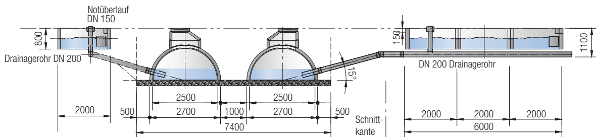
Versickerungsanlage Innodrain
