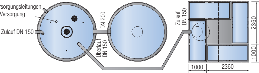
Regenspeicher B mit 2 Filterkörben 2-Behälteranlage
