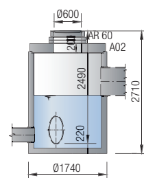
Vereinigungsbauwerk ViaPool
