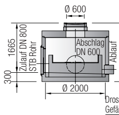
Trennbauwerk ViaSep
