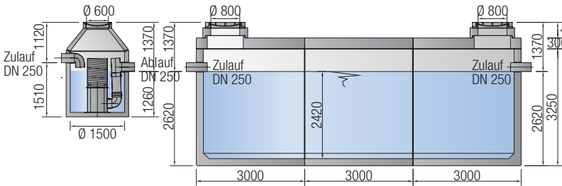
Filterschacht
