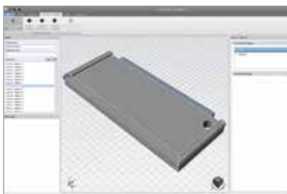
Berücksichtigung von Aufkantungungen oder Aussparungen in der Balkonplatte
