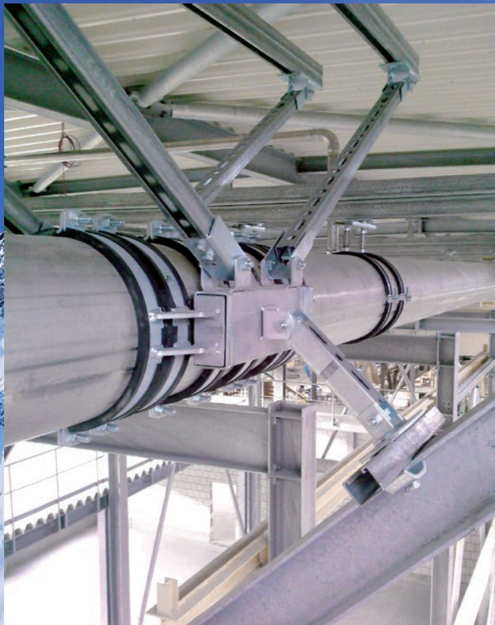
Festpunktlösungen für verschiedene Rohrtypen
