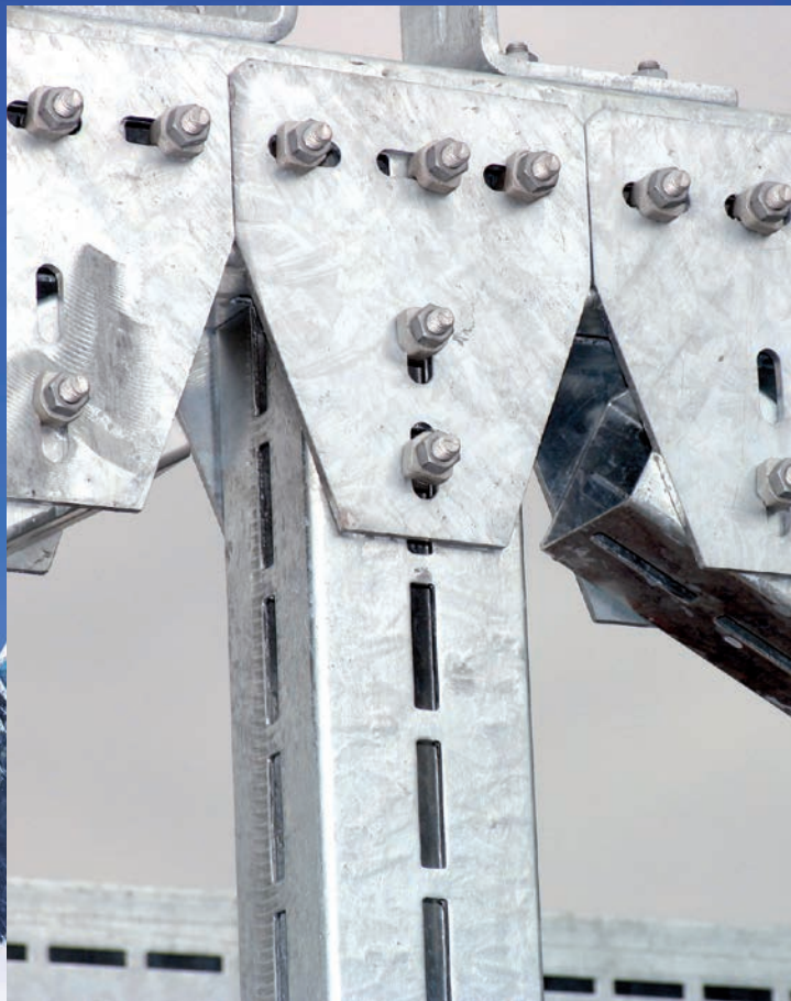
RLT-Anlage auf Dachkonstruktion CENTUM® Schwerlastsystem mit Anbauteilen
