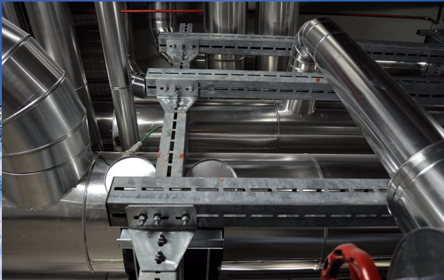
Halterung über mehrere Etagen Schwerlast CENTUM® mit gewinkelten T-Laschen
