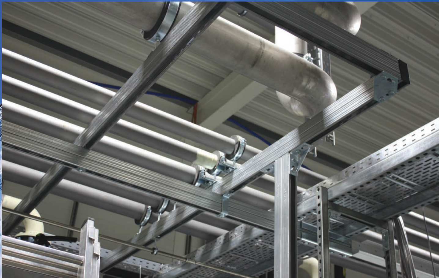
Stützkonstruktion für Kälterohrleitungen Montageschienen System 45/90 mit Kälteschelle Polar plus
