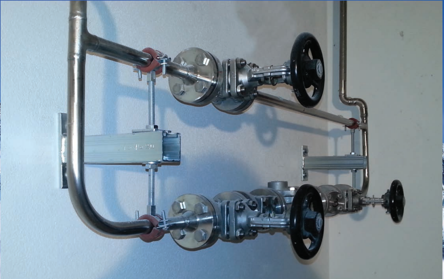
Konsolenhalterung für Absperrhähne Konsole 45/45/2,0 längs
