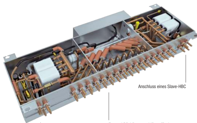
Zu- und Rückflussanschlüsse für das Wassersystem; es sind Ausführungen mit 8 oder 16 Anschlüssen erhältlich.
