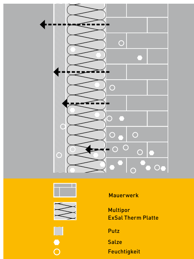
Prinzipiskizze
