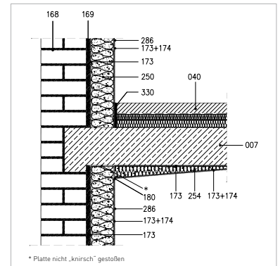
Stahlbetondecke mit Dämmkeil/ Außenwand mit Innendämmung
