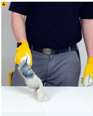
4 Leichtmörtel auftragen
