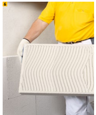
6 Mörtel vollflächig auf Mineraldämmplatte
