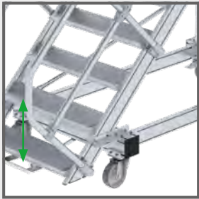
ZBS 2-4 Vier Lenkrollen durch Fuß-Bedienhebel bedienbar
