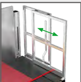
Schiebegeländer ausgefahren
