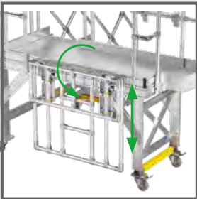
Geländer absenkbar und klappbar (Darst. untere Stellung)
