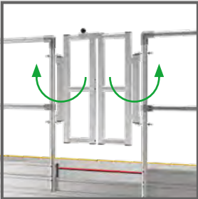
Doppelflügel Sicherheitstüre mit Überwurfbügel
