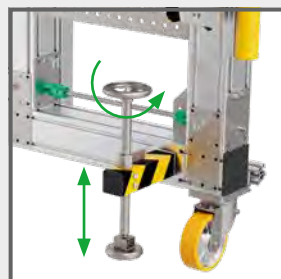
Stützspindel für erhöhte Standsicherheit
