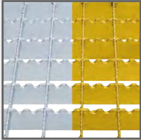
Stufenbelag R12 Stahl-Gitterrost oder gelb beschichtet
