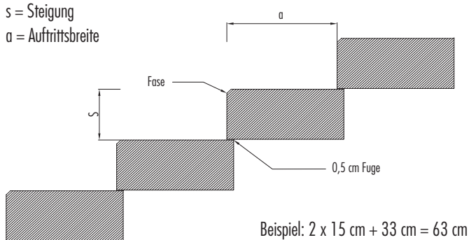
Steigungsprinzip Treppe
