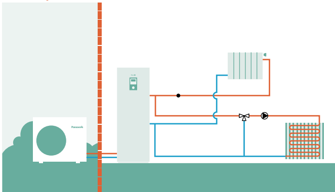
Aquarea J- und H-Generation: Zwei Heizkreise mit Aquarea Kombi-Hydrmodul, ohne Pufferspeicher
