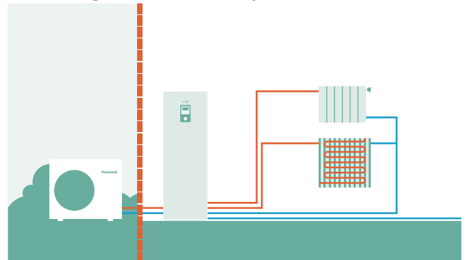
Aquarea J- und H-Generation: Zwei Heizkreise mit Aquarea Kombi-Hydrmodul in Ausführung „B“ 1 , ohne Pufferspeicher
