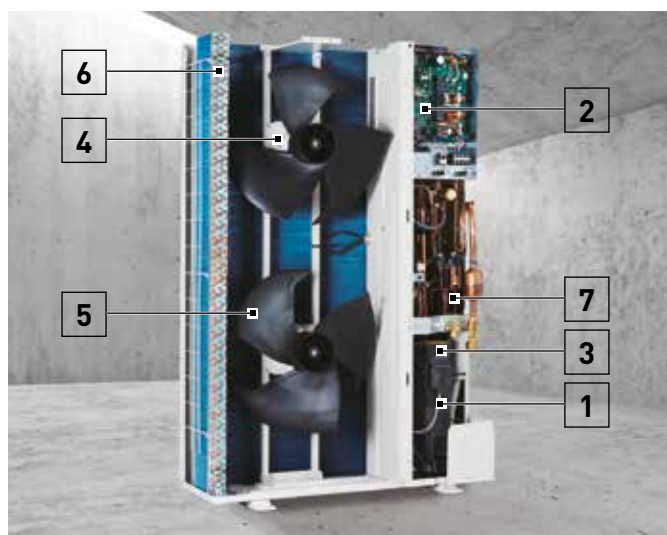
Leistungstarker Wärmeübertrager Kompakter dreilagiger Wärmeübertrager: Trotz des um 15 % kleineren Gerätegehäuses bei den einphasigen 4-, 5- und 6-PS-Geräten ist die Oberfläche des neuen Wärmeübertragers genau so groß wie bei den Vorgängermodellen.
