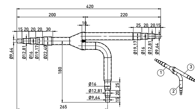
Flüssigkeitsleitung
