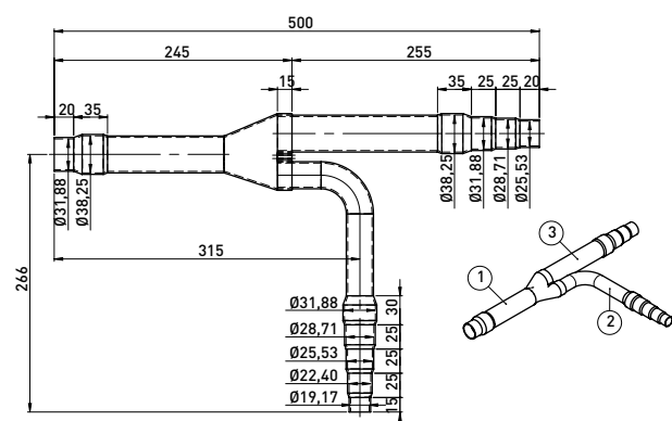
Gasleitung
