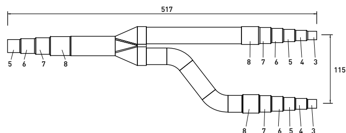
Gasleitung
