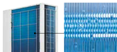
Wärmeübertrager (Verflüssiger mit Bluefin-Antikorrosionsbeschichtung)
