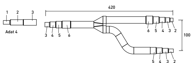
Flüssigkeitsleitung
