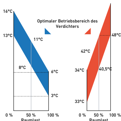
Verdampfungstemperatur Verflüssigungstemperatur
