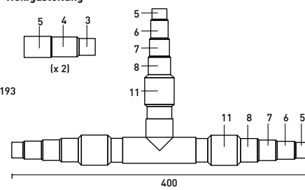
Heißgasleitung
