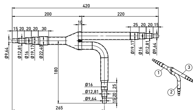
Flüssigkeitsleitung
