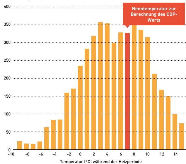
Zeitliche Verteilung der Außentemperatur
