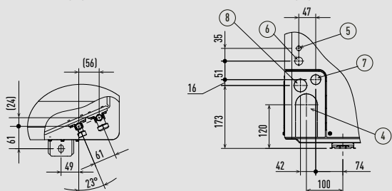
Ansicht A
