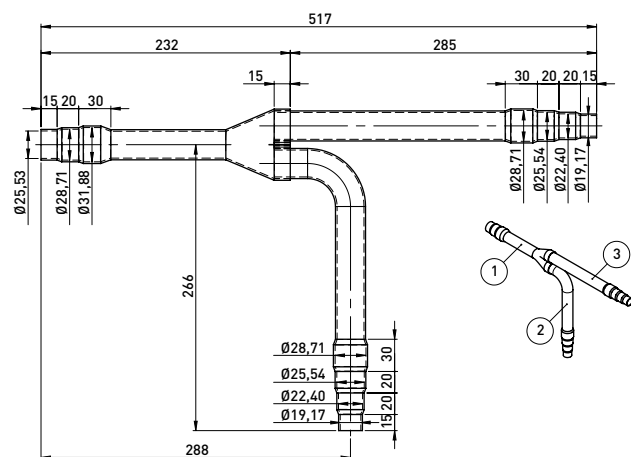
Gasleitung
