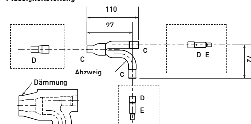
Flüssigkeitsleitung
