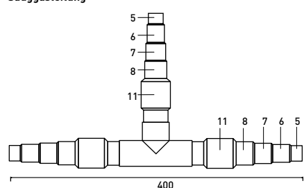
Sauggasleitung
