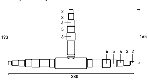
Flüssigkeitsleitung
