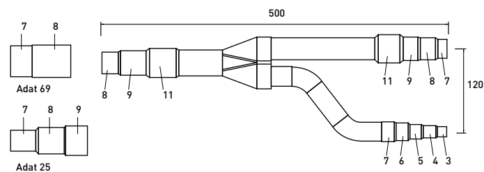
Gasleitung
