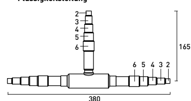
Flüssigkeitsleitung
