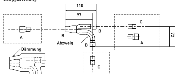
Sauggasleitung
