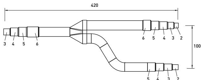
Gasleitung
