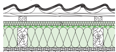
Abb.16 Konstruktionsbeispiel
