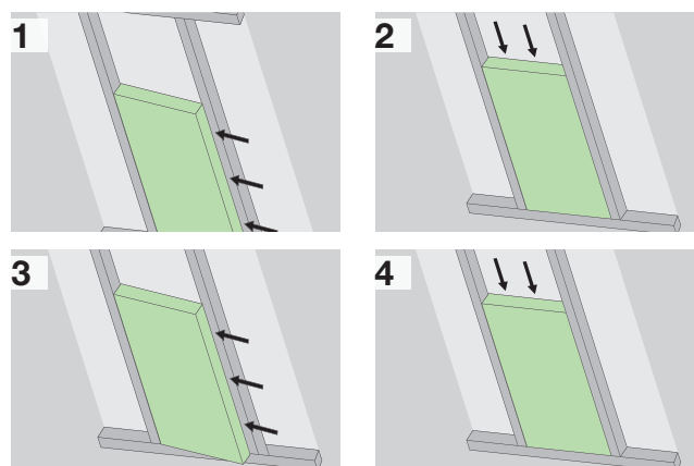
Abb.17 Verlegeprinzip PAVAFLEX CONFORT 36 (schematische Darstellung)
