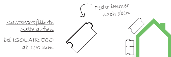
Abb.12 Profilierung ISOLAIR ECO ab 100 mm
