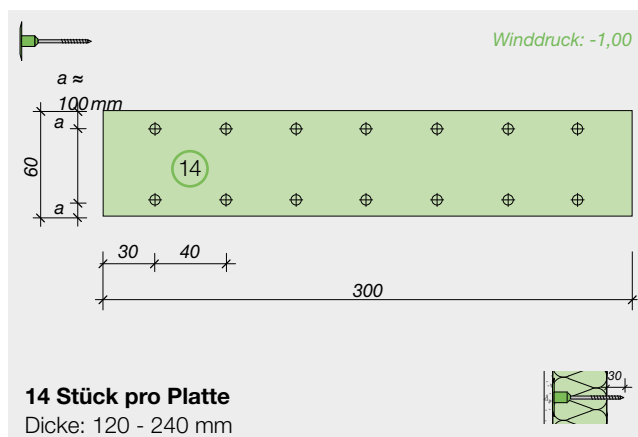
Schemazeichnung
