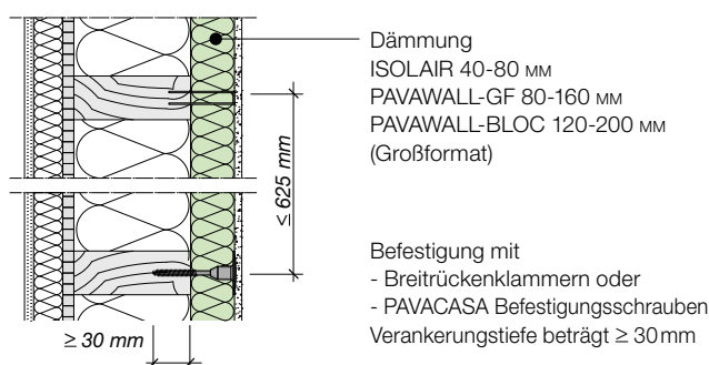
Abb. 6 Befestigungsmittel
