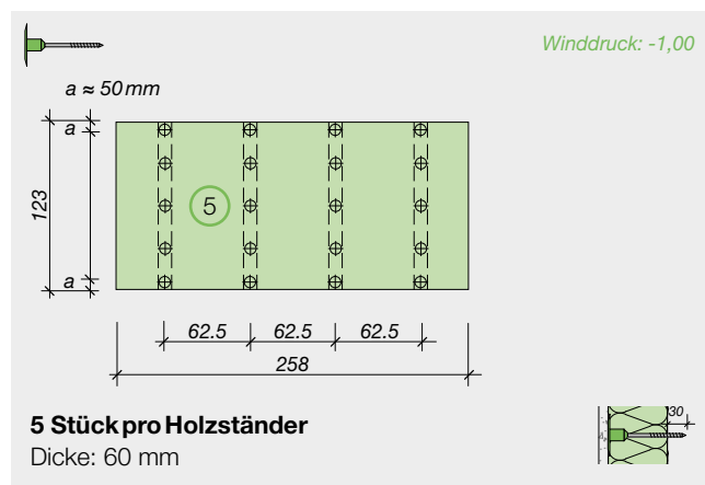
Schemazeichnung
