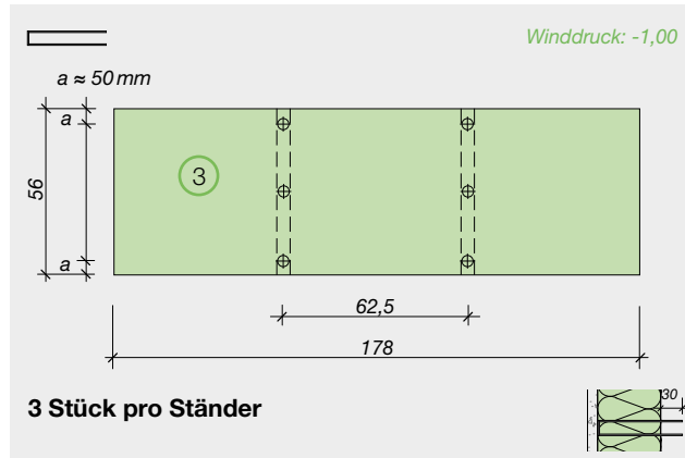
Schemazeichnung
