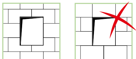
Abb. 4 Fenster-Türöffnungen mit Ausklinkung
