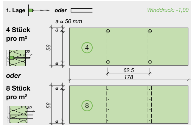
Schemazeichnung
