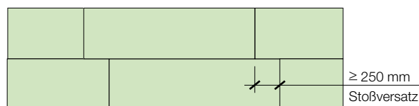
Abb. 3 Stoßversatz bei der Verlegung von ISOLAIR, PAVAWALL-GF und PAVAWALL-BLOC (Großformat)
