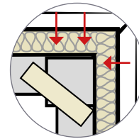
Fuge umlaufend hohlraumfrei mit Dämmstoff ausfüllen
