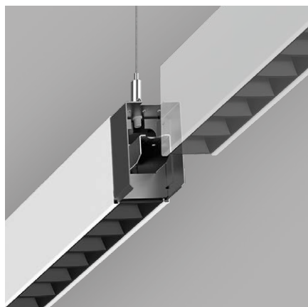
Einfacher Aufbau eines Pendel-Lichtbandes.
