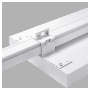
Tragschienenmontage mit Befestigungsbügel BW-SDT
