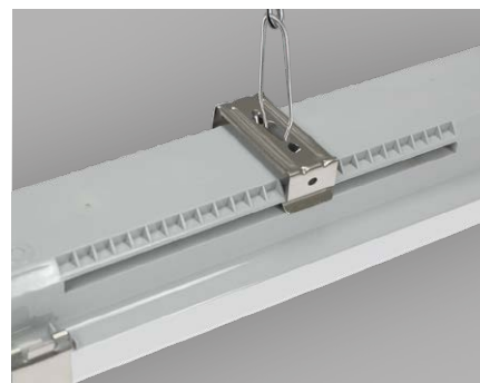
Edelstahl Universal-Befestigungs-Clips sowie Abhängbügel im Lieferumfang
