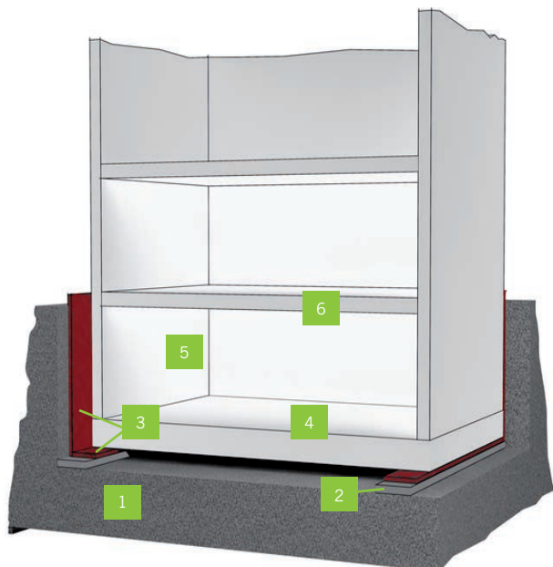
Streifenförmige Entkopplung eines Gebäudefundamentes mit Regupol®/Regufoam® Schwingungsdämmmaterial: 1 Natürlicher Untergrund • 2 Impedanzplatte • 3 Regupol®/Regufoam® Schwingungsisolierung • 4 Fundamentplatte • 5 Kellerwand • 6 Geschossdecke
