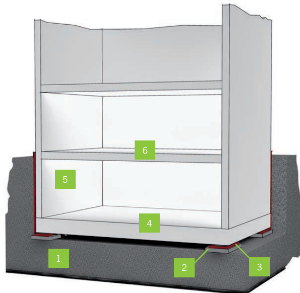
Punktuelle Entkopplung eines Gebäudefundamentes mit Regupol®/Regufoam® Schwingungsdämmmaterial: 1 Natürlicher Untergrund • 2 Impedanzplatte • 3 Regupol®/Regufoam® Schwingungsisolierung • 4 Fundamentplatte • 5 Kellerwand • 6 Geschossdecke
