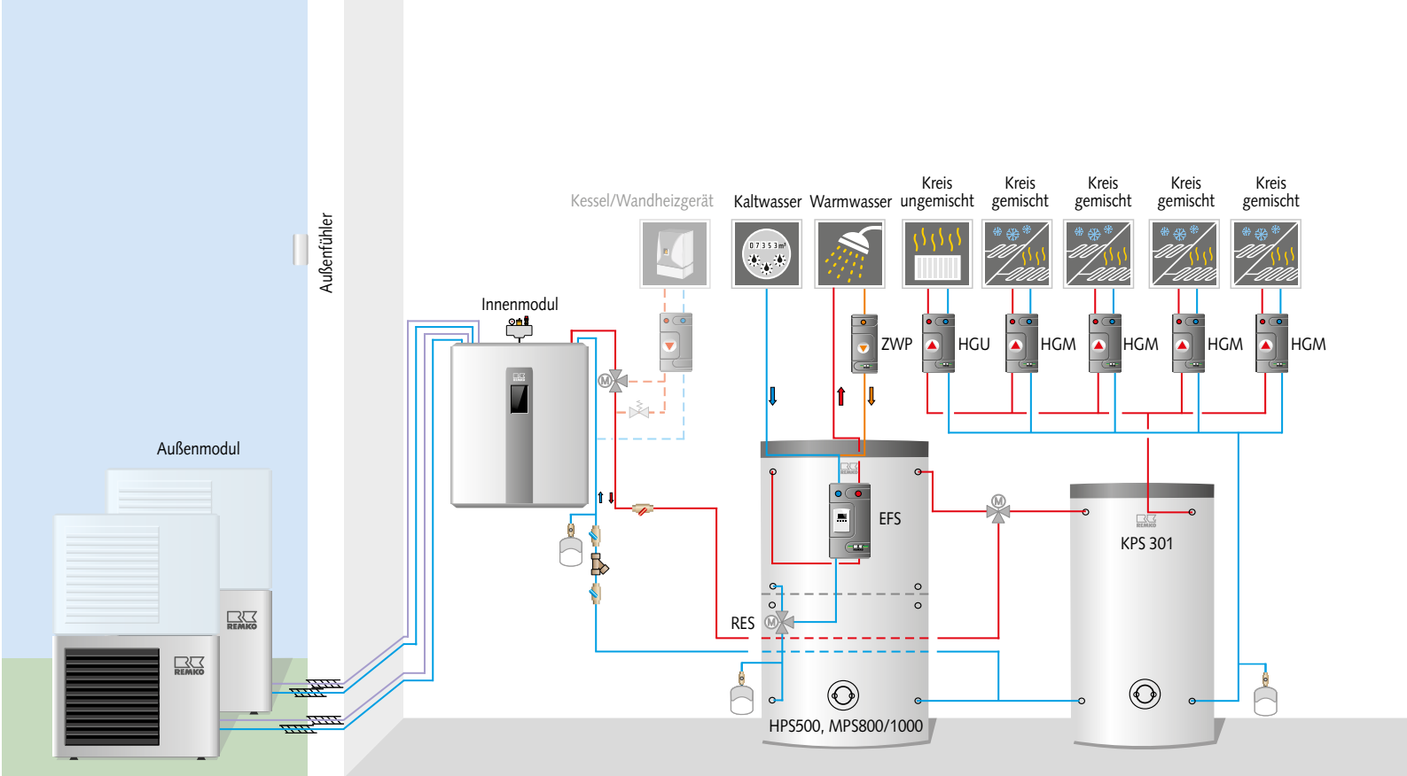
Hydraulischeschema München Duo (Beispiel für monoenergetische oder bivalent alternative Betriebsart)
