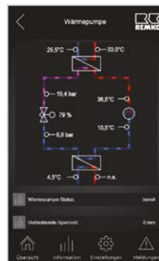
Darstellung Kältekreislauf
