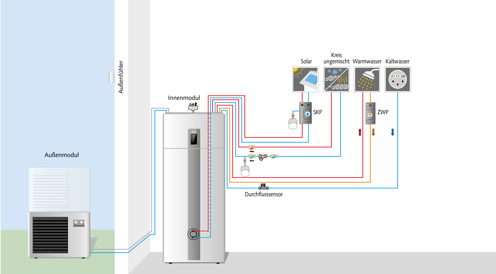
Hydraulischeschema Stuttgart Solar (Beispiel für monoenergetische Betriebsart und solarunterstützte Trinkwasserbereitung)
