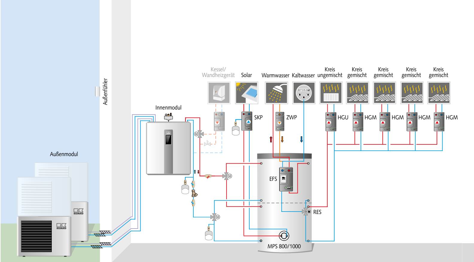
Hydraulikschema Frankfurt Duo/ Frankfurt Duo Solar (Beispiel für monoenergetische oder bivalent alternative Betriebsart)
