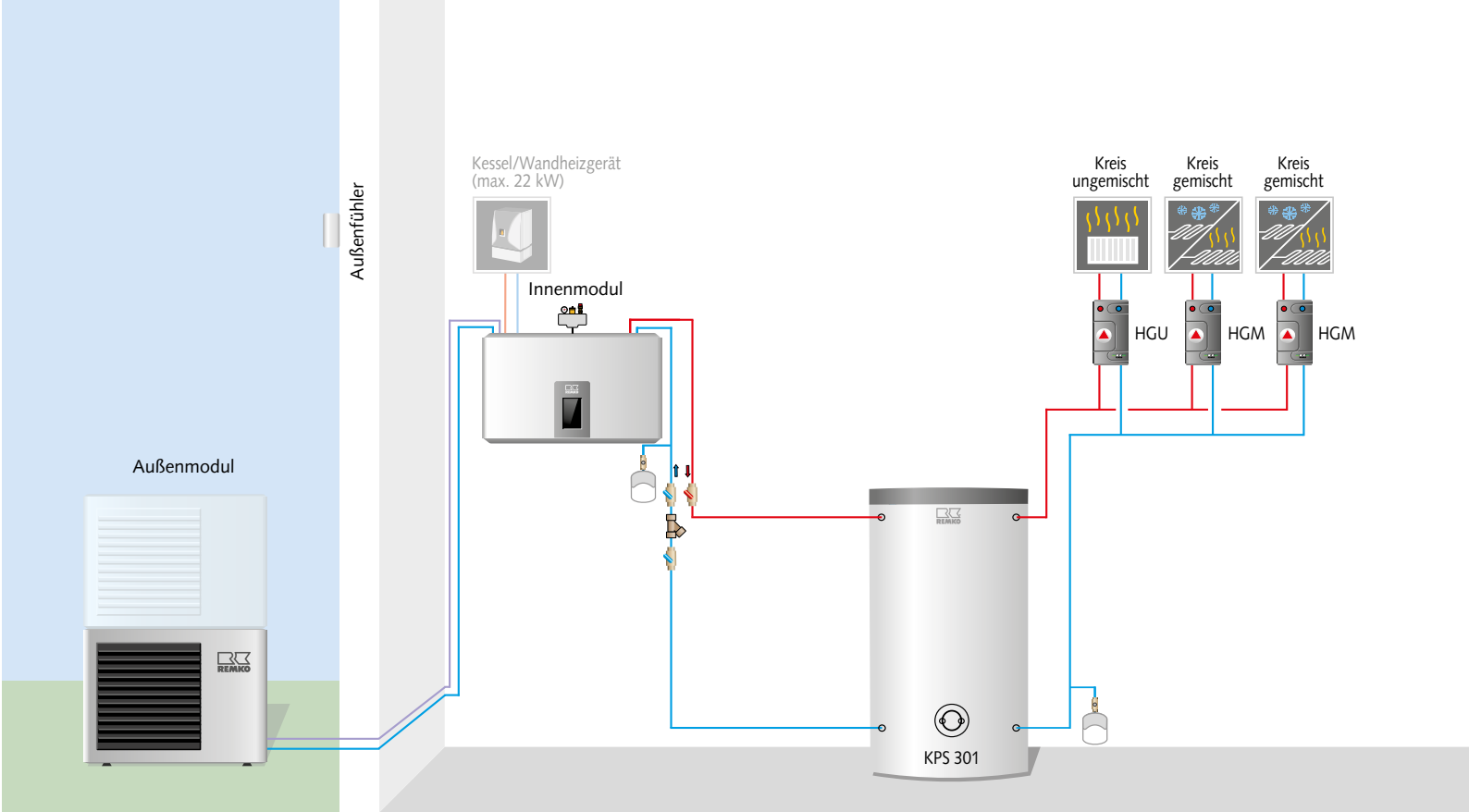
Hydraulikschemata Köln (Beispiel für monoenergetische oder bivalent alternative Betriebsart)
