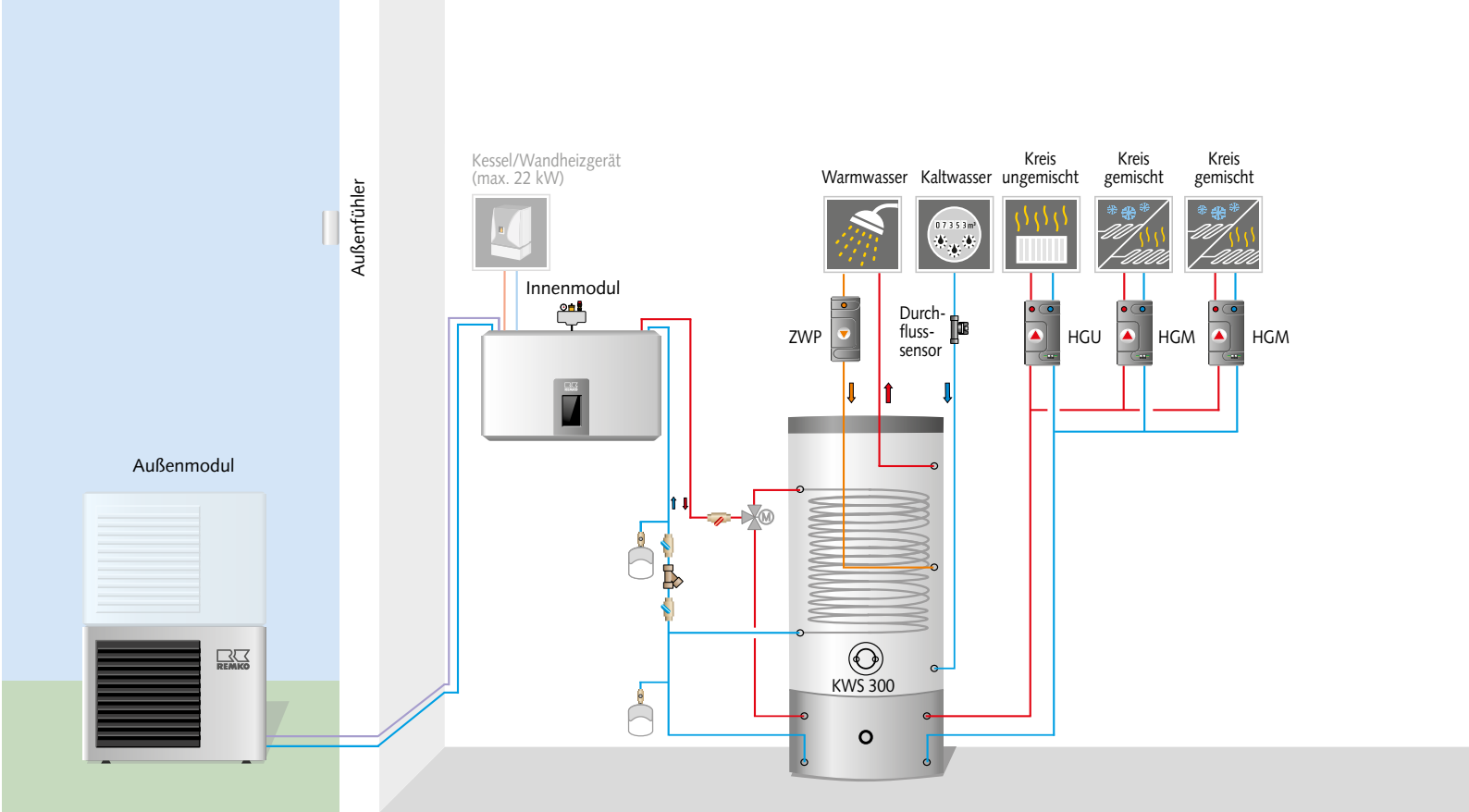
Hydraulischeschema Mannheim (Beispiel für monoenergetische oder bivalent alternative Betriebsart)
