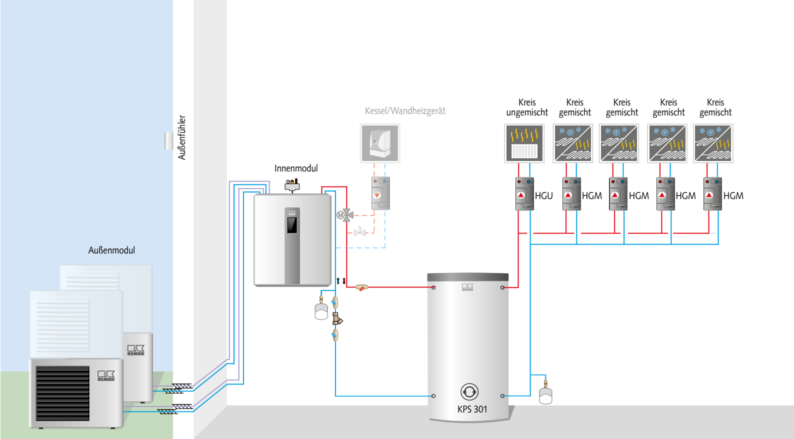
Hydraulikschemata Köln Duo (Beispiel für monoenergetische oder bivalent alternative Betriebsart)
