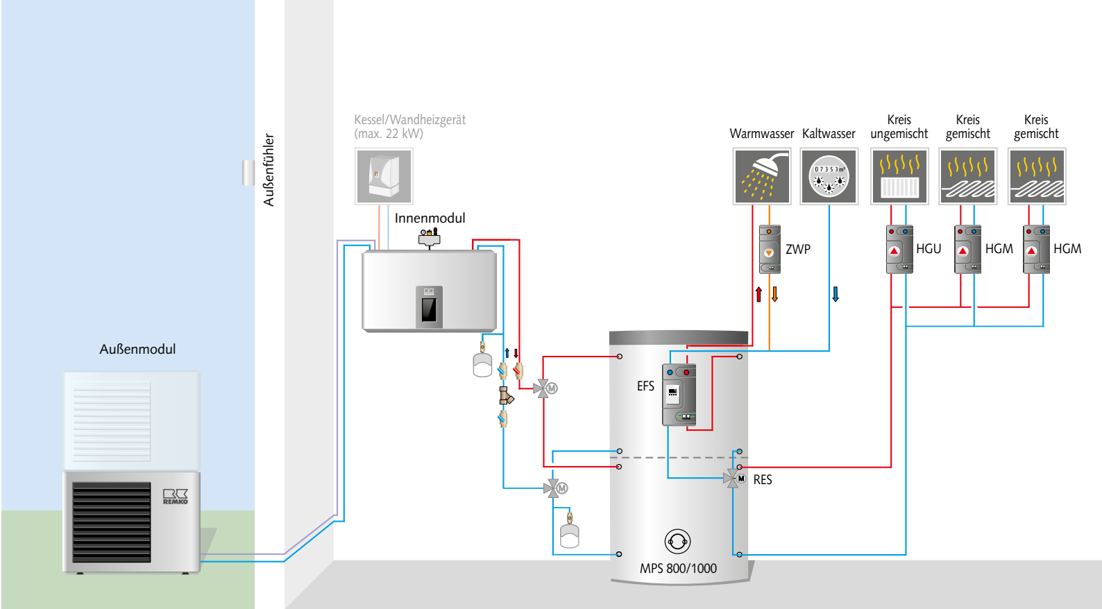
Hydraulikschemata Frankfurt (Beispiel für monoenergetische oder bivalent alternative Betriebsart)
