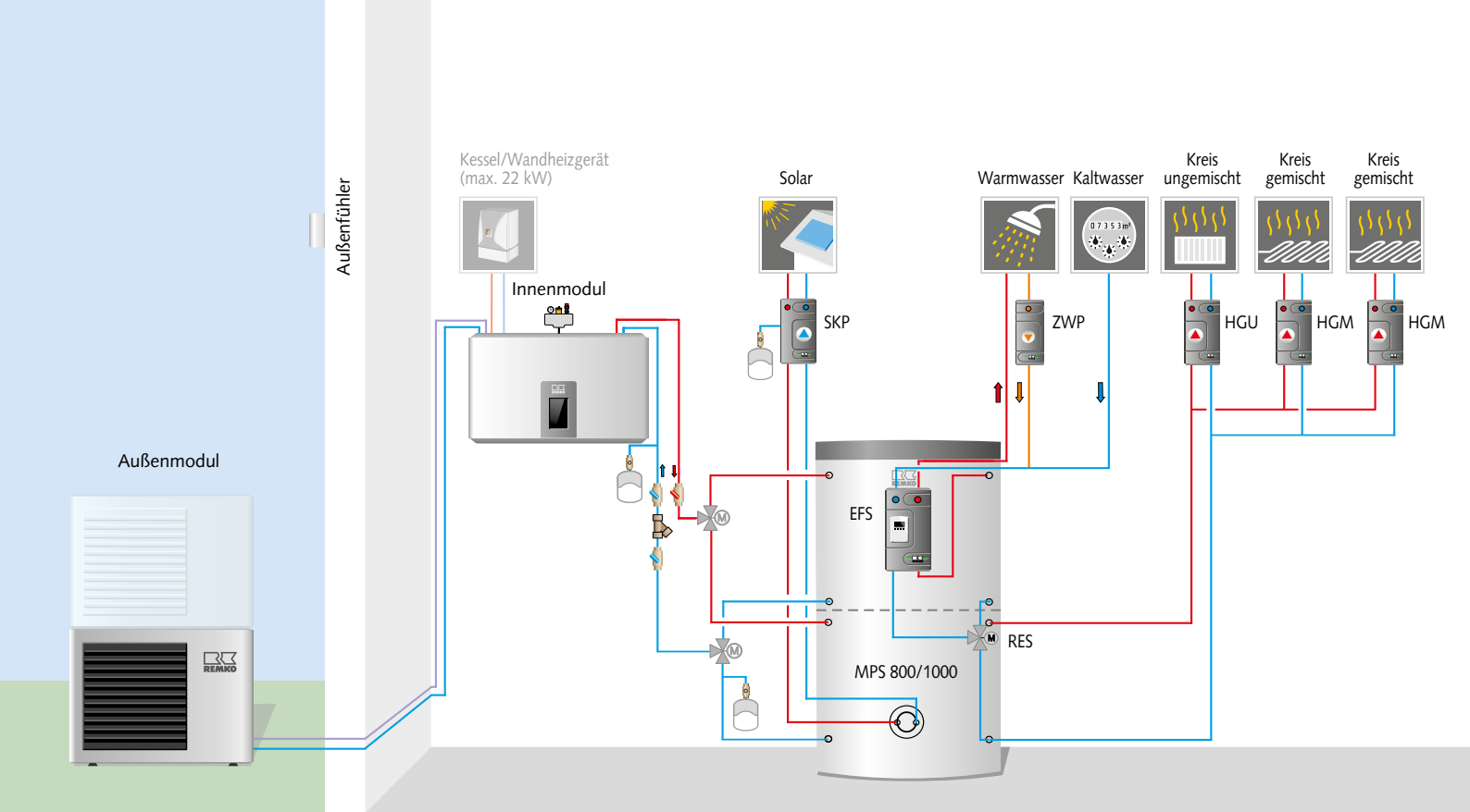
Hydraulischeschema Frankfurt Solar (Bsp. für monoenergetische oder bivalent alternative Betriebsart und solarunterstützte Heizung/Trinkwasserbereitung)
