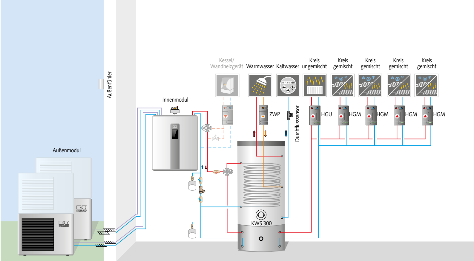
Hydraulischeschema Mannheim Duo (Beispiel für monoenergetische oder bivalent alternative Betriebsart)
