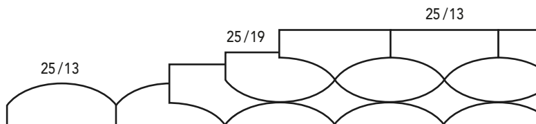
Kettengebinde Nr. 4 = 16 Steine
